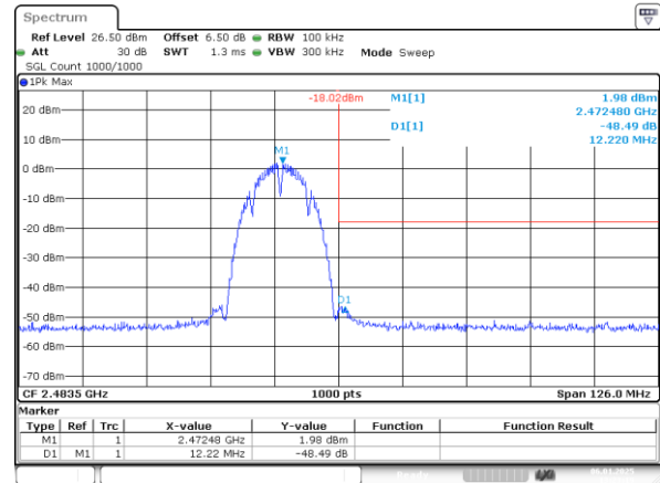
802.11b_2472MHz
