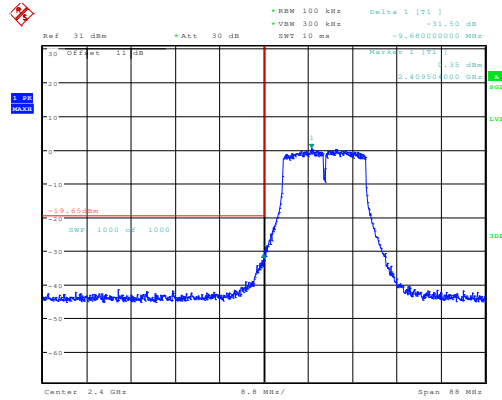
802.11g_2412MHz 31.50dB
