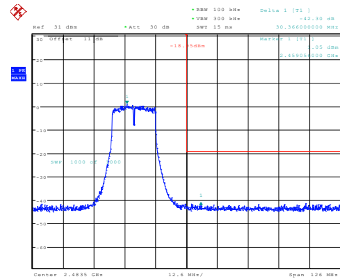
802.11n20_2462MHz 42.30dB
