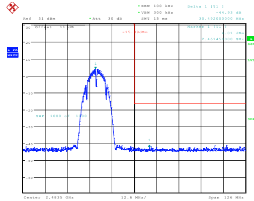
802.11b_2462MHz 44.93dB
