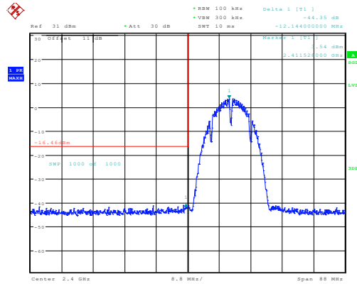
802.11b_2412MHz 44.35dB
