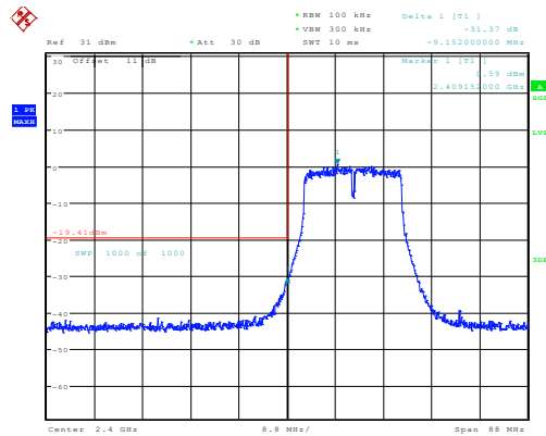
802.11n20_2412MHz 31.37dB
