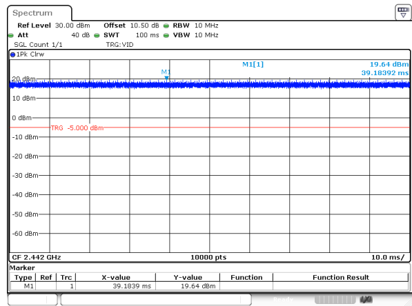
802.11n20_2442MHz
