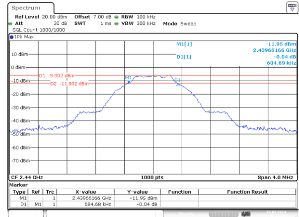
Middle 0.685MHz
