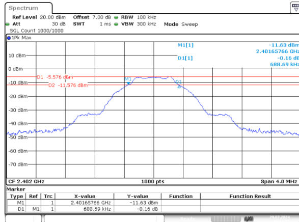
Low 0.689MHz
