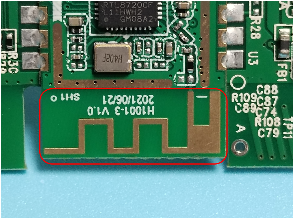
Wi-Fi ANT
