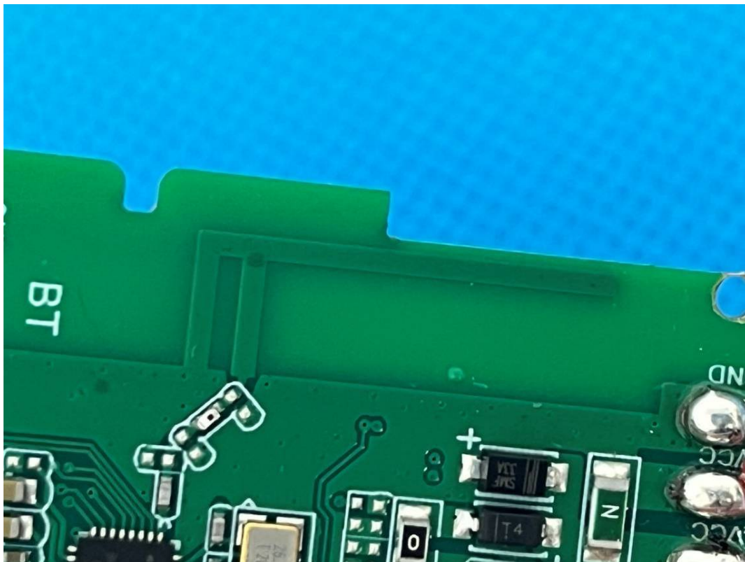
BLE ANT
