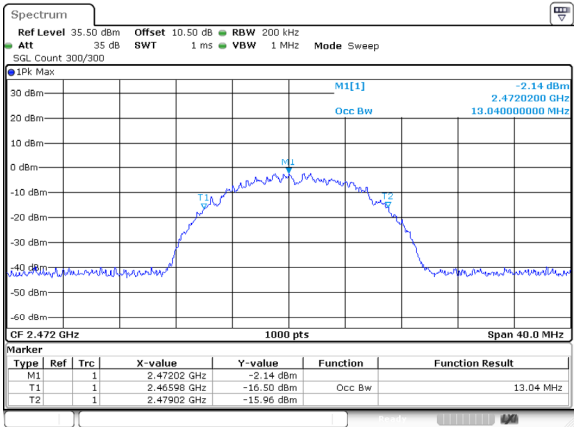
802.11b_2472MHz
