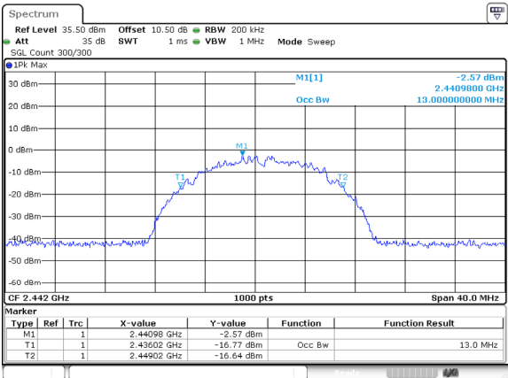
802.11b_2442MHz
