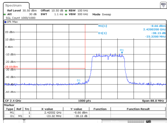
802.11n20_2412MHz
