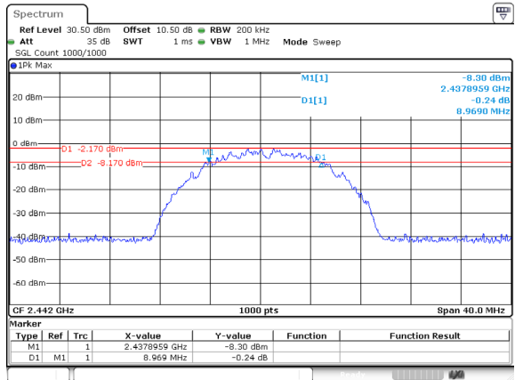
802.11b_2442MHz
