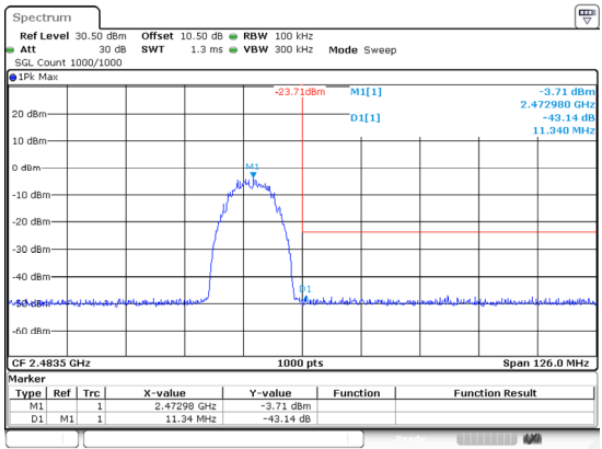
802.11b_2472MHz
