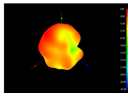
2500MHz
