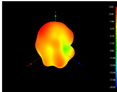
2400MHz
