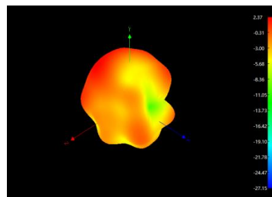
2450MHz
