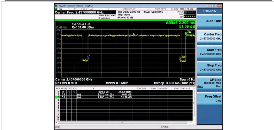
NTNV-11G-Ant1-2437
