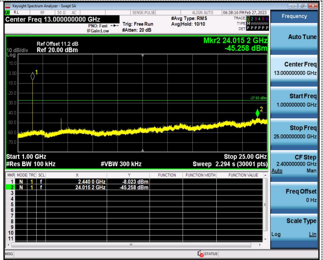
1G-25G
