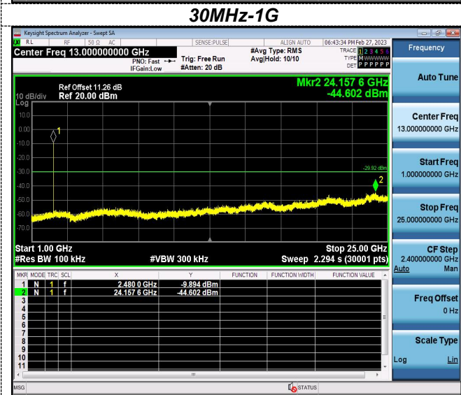
1G-25G
