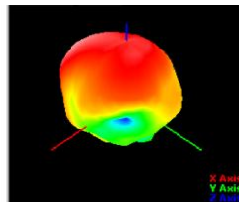
2465MHz
