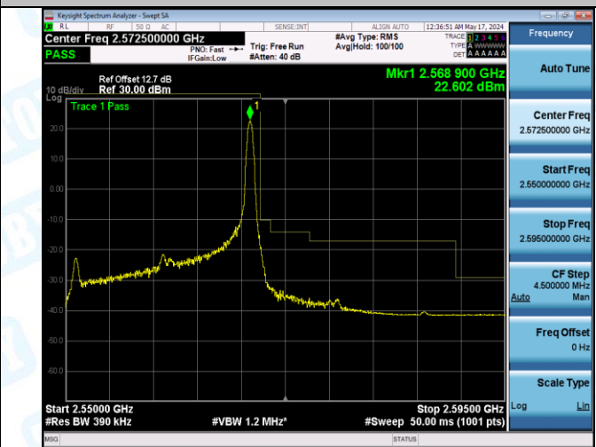
Band7_20MHz_16QAM_21350_1RB#99
