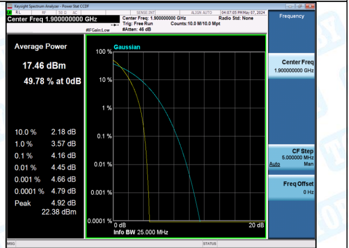
Band2-20MHz-16QAM-18700-27RB#0-PASS
