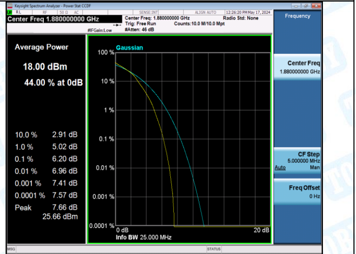
Band2-20MHz-16QAM-19100-27RB#0-PASS
