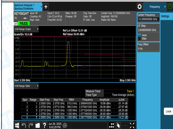
Band7-20MHz-QPSK-21350-1RB#99-PASS
