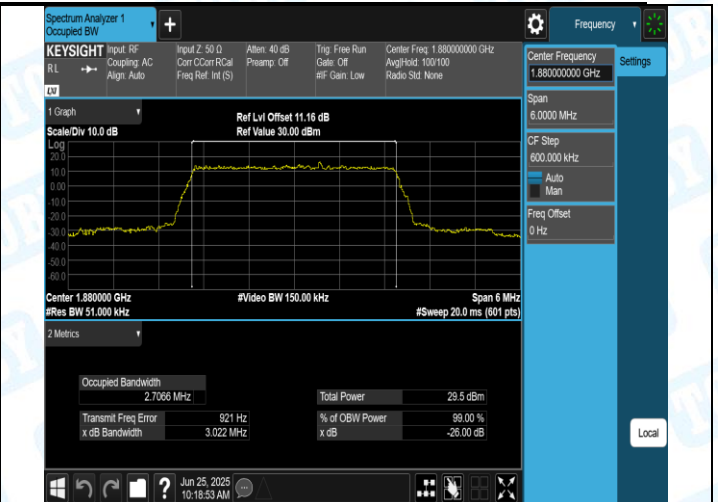
Band2-3MHz-QPSK-18900-15RB#0-PASS
