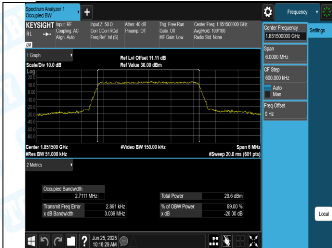
Band2-3MHz-QPSK-18615-15RB#0-PASS
