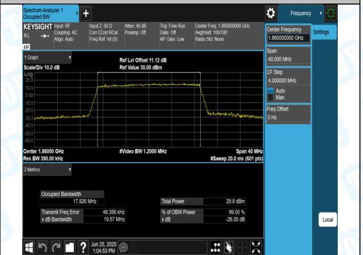
Band2-20MHz-16QAM-18700-100RB#0-PASS
