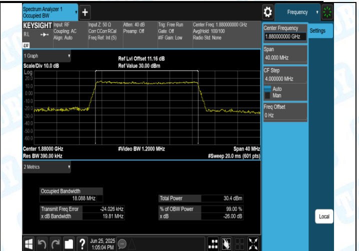
Band2-20MHz-QPSK-18900-100RB#0-PASS
