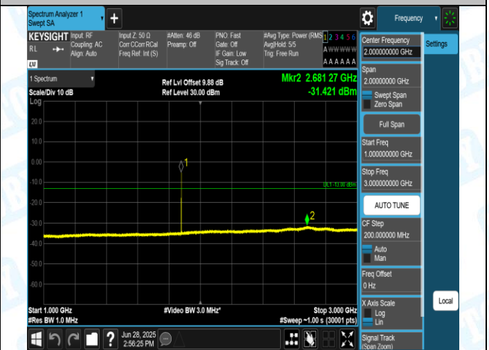
GPRS1900-661-0-1000~3000MHz-PASS
