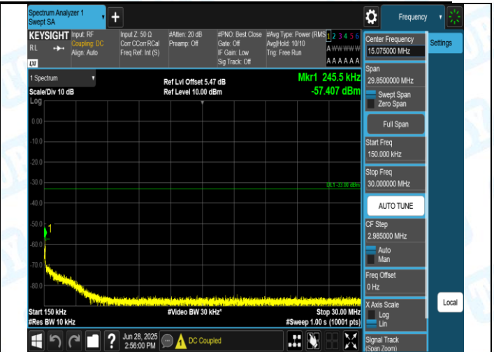
GPRS1900-661-0-0.15~30MHz-PASS
