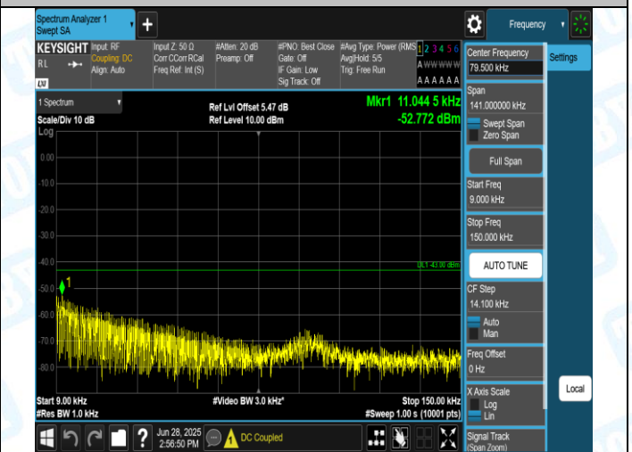
GPRS1900-810-0-0.009~0.15MHz-PASS
