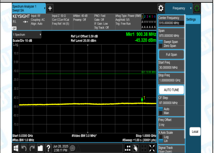
GPRS1900-661-0-30~1000MHz-PASS
