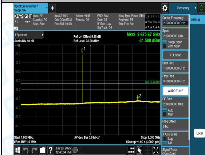
GSM1900-661-0-1000~3000MHz-PASS
