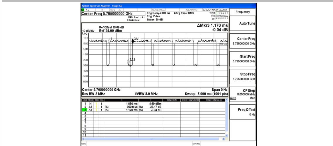
NTNV-11N40MIMO-Ant1-5795
