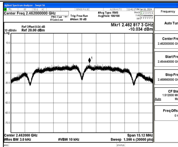
11B-Ant2-2462-PASS
