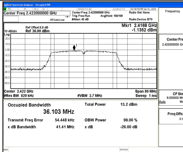
11N40MIMO-Ant1-2422
