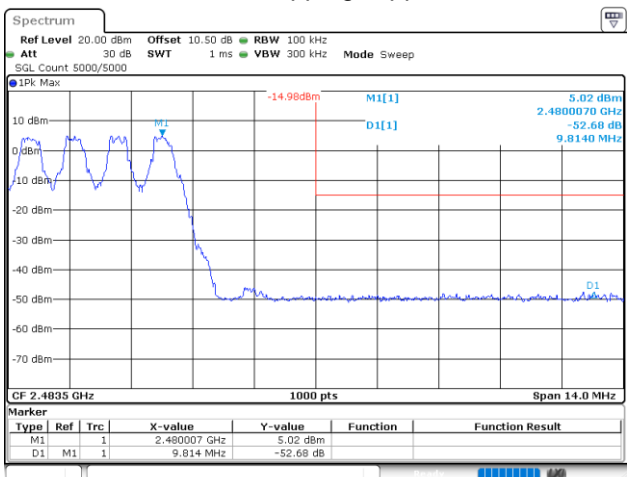
DH1_Hopping_Upper
