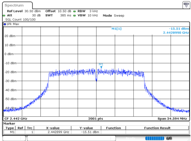
802.11n20_2442MHz_Chain 0
