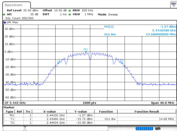
802.11b_2442MHz_Chain 0
