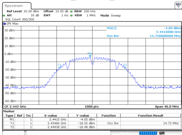
802.11b_2442MHz_Chain 1
