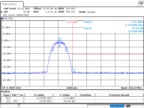
802.11b_2472MHz_Chain 0
