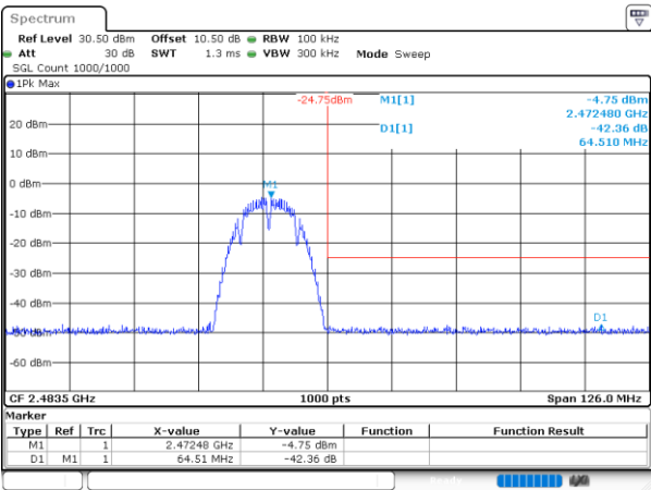
802.11b_2472MHz_Chain 1
