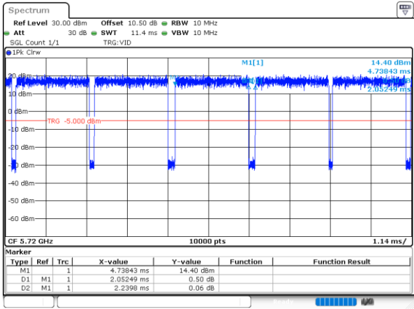
802.11a_5720MHz_Chain 0
