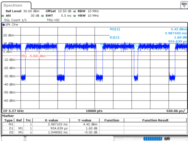
802.11n40_5270MHz_Chain 1
