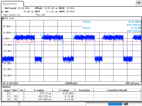
802.11ac80_5290MHz_Chain 1
