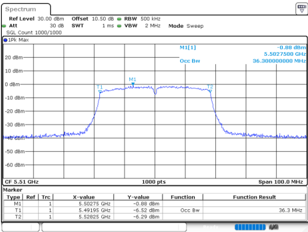
802.11n40_5510MHz_Chain 1
