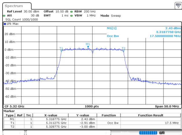
802.11n20_5320MHz_Chain 0
