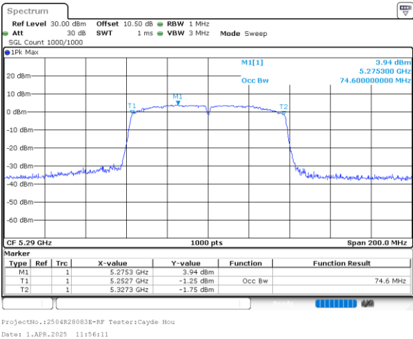
802.11ac80_5290MHz_Chain 0
