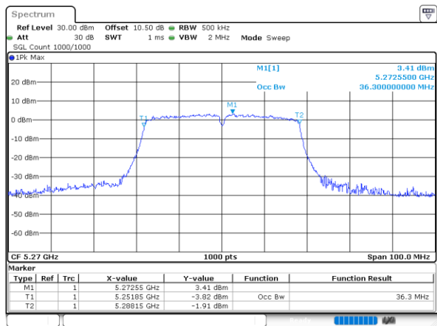
802.11n40_5270MHz_Chain 0
