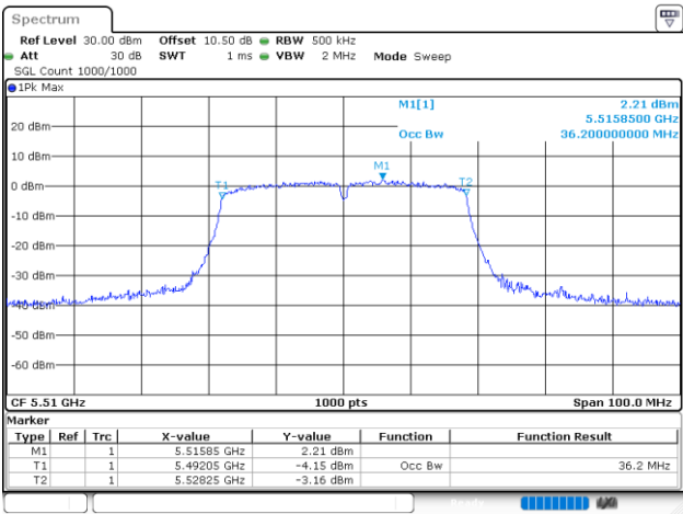
802.11n40_5510MHz_Chain 0
