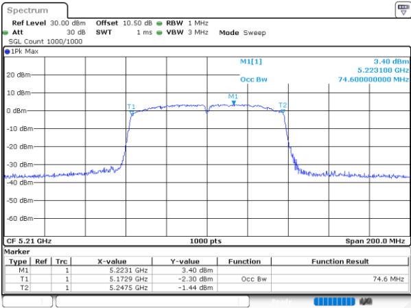
802.11ac80_5210MHz_Chain 0
