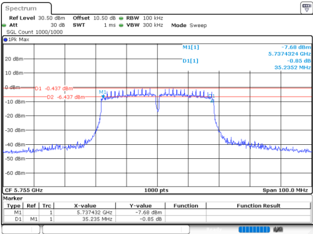
802.11n40_5755MHz_Chain 1
