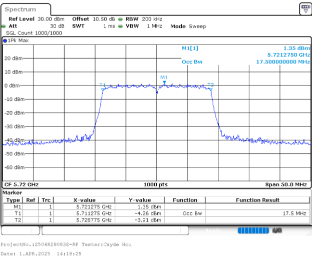
802.11n20_5720MHz_Chain 1
