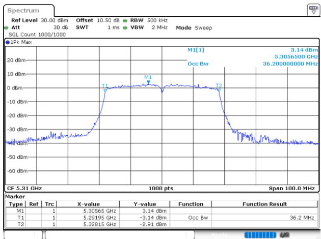
802.11n40_5310MHz_Chain 0
