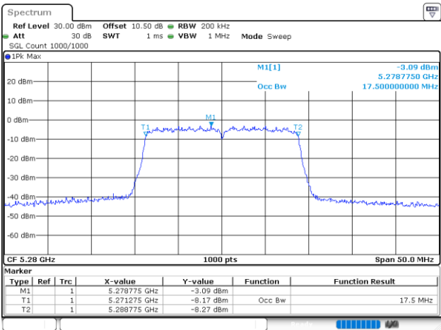
802.11ac20_5280MHz_Chain 1
