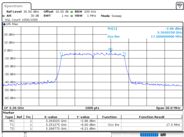
802.11n20_5260MHz_Chain 1
