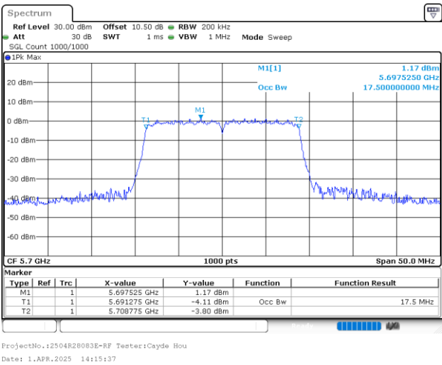
802.11n20_5700MHz_Chain 1
