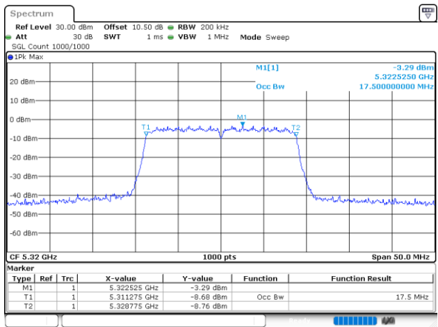
802.11n20_5320MHz_Chain 1
