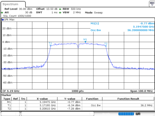
802.11ac40_5190MHz_Chain 1
