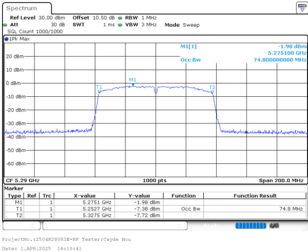
802.11ac80_5290MHz_Chain 1
