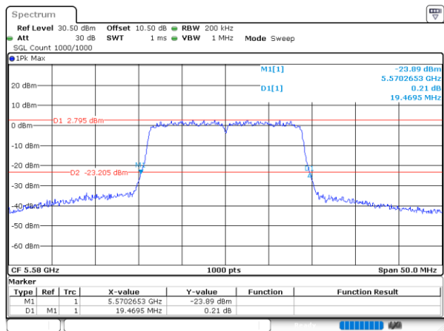
802.11n20_5580MHz_Chain 0
