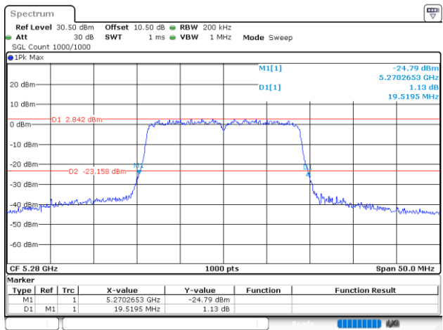
802.11ac20_5280MHz_Chain 0
