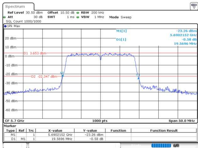
802.11n20_5700MHz_Chain 0
