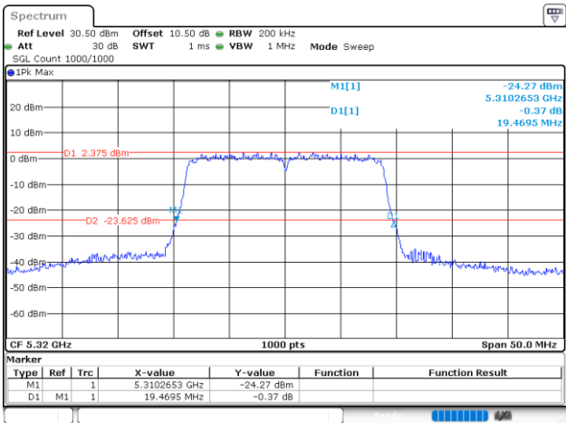
802.11n20_5320MHz_Chain 0
