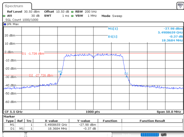
802.11a_5500MHz_Chain 1
