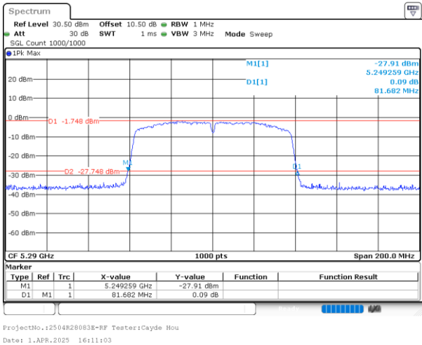
802.11ac80_5290MHz_Chain 1
