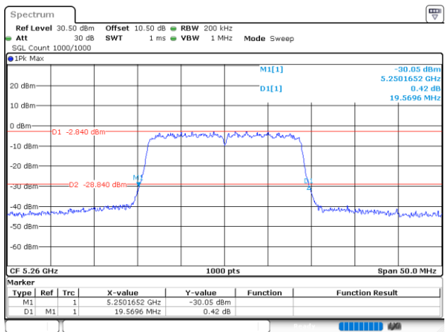
802.11ac20_5260MHz_Chain 1
