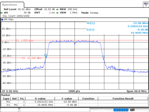
802.11ac20_5260MHz_Chain 0
