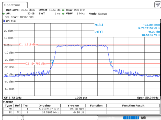
802.11a_5720MHz_Chain 1
