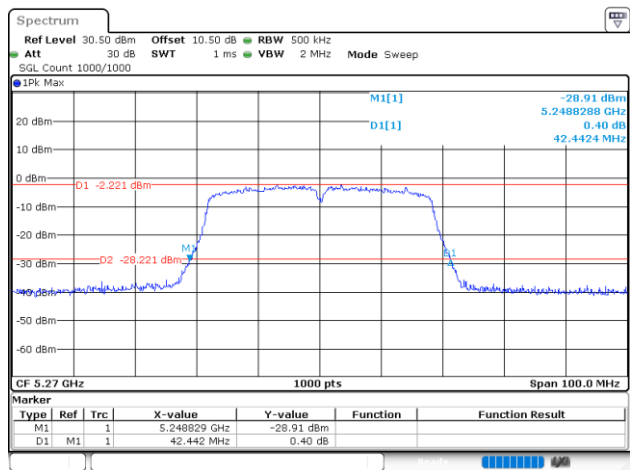
802.11n40_5270MHz_Chain 1
