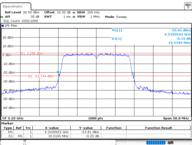
802.11ac20_5320MHz_Chain 0
