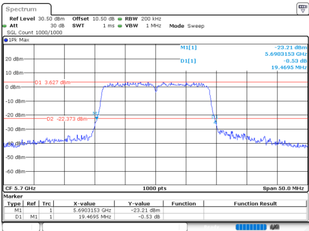
802.11ac20_5700MHz_Chain 0
