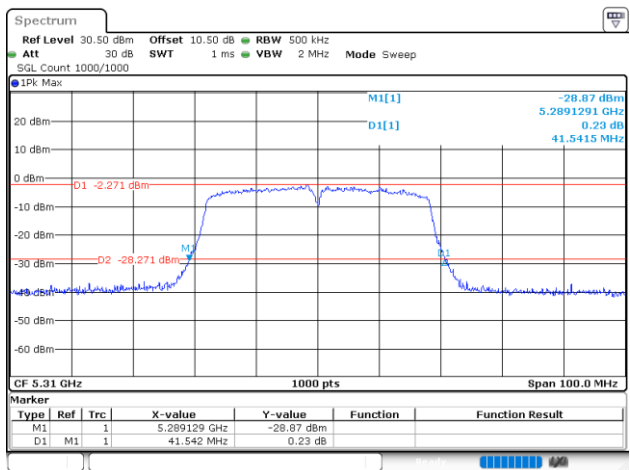
802.11n40_5310MHz_Chain 1
