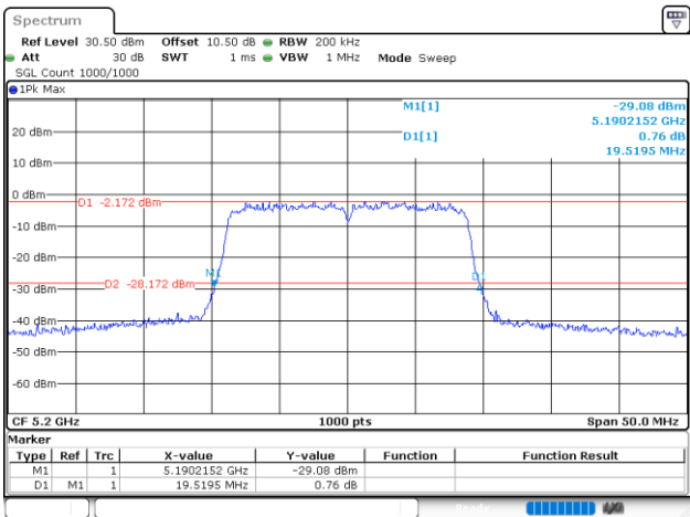
802.11n20_5200MHz_Chain 1
