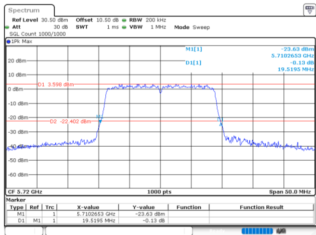
802.11n20_5720MHz_Chain 0
