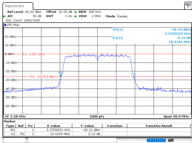
802.11n20_5580MHz_Chain 1
