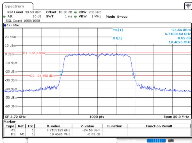
802.11n20_5720MHz_Chain 1
