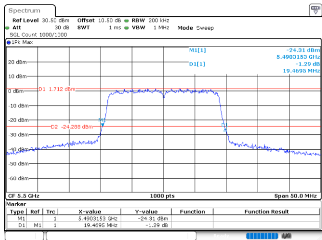
802.11n20_5500MHz_Chain 0
