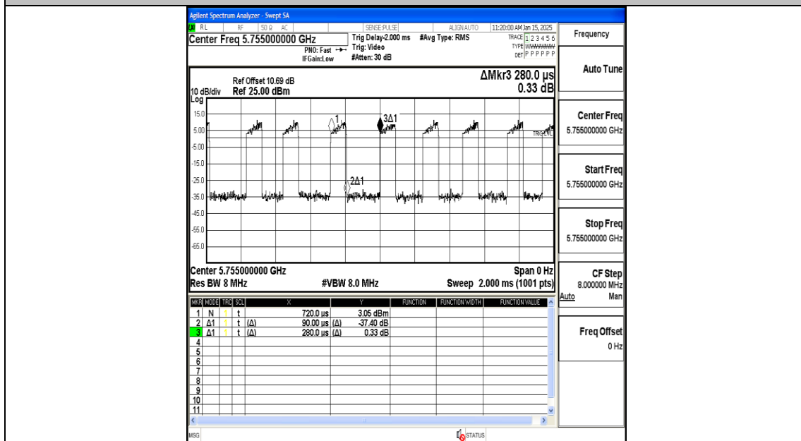
NTNV-11N40MIMO-Ant1-5755
