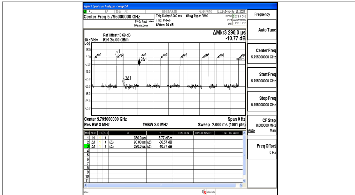
NTNV-11N40MIMO-Ant1-5795
