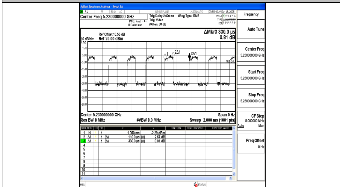
NTNV-11AC40MIMO-Ant1-5230
