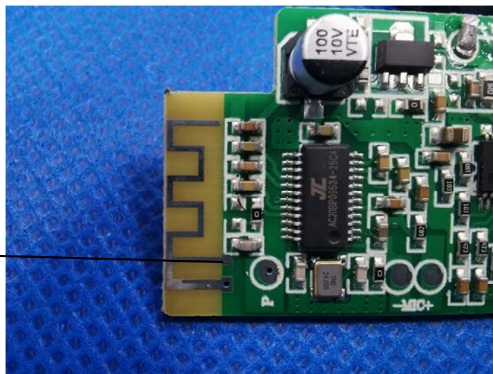
BLE Antenna
