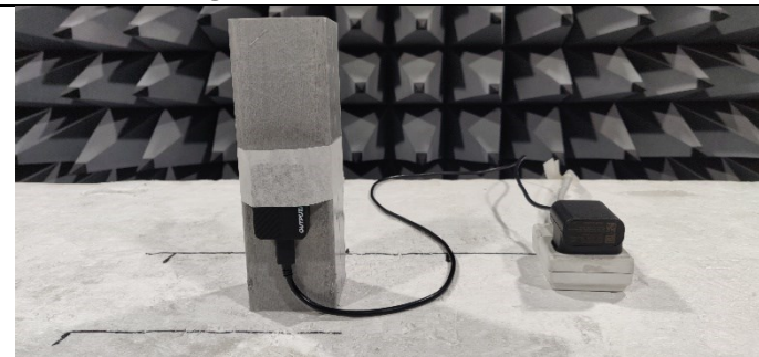
Fig B7: EUT Close up
