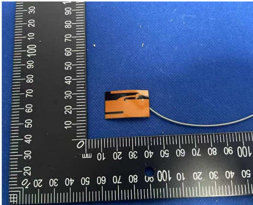
EUT Photo
