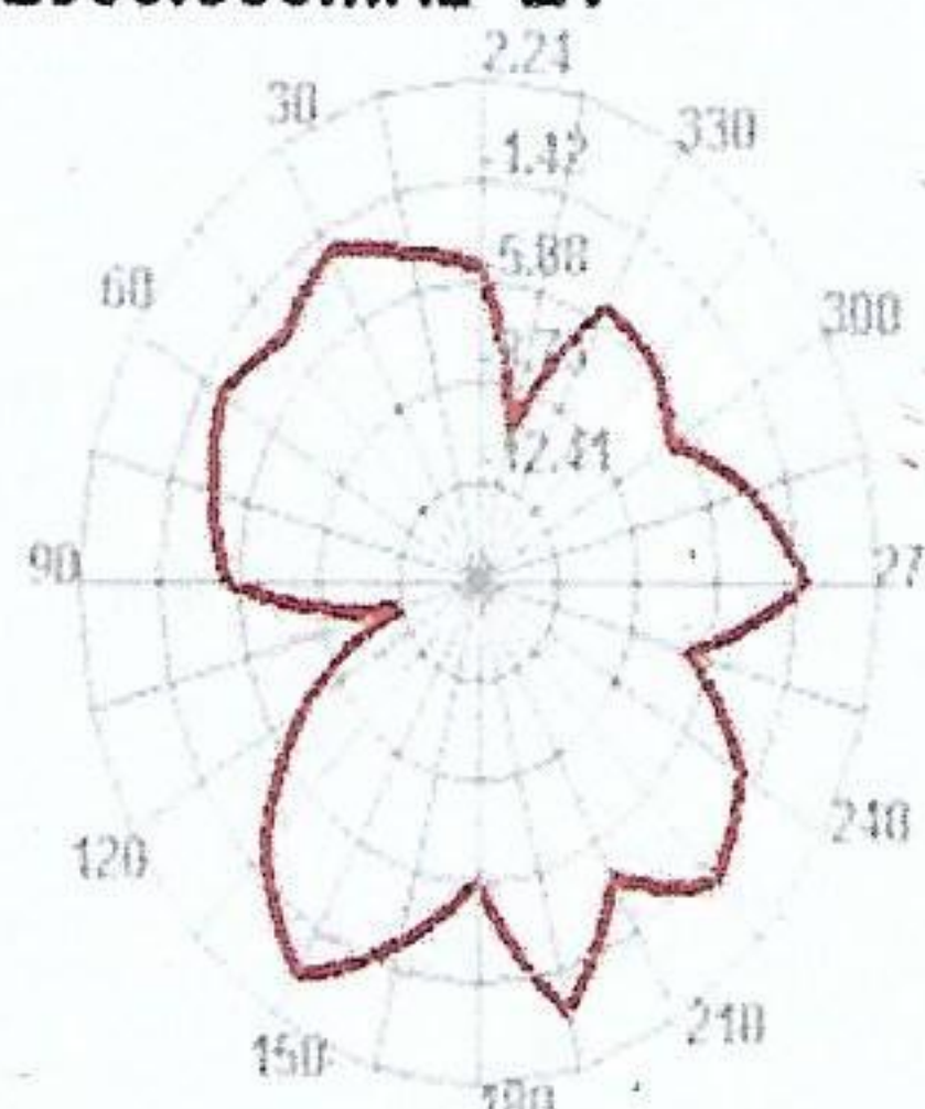
2500.000MHz E1
