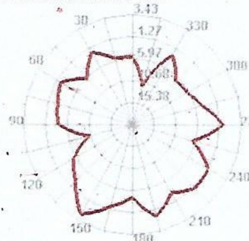
2450.000MHz E1
