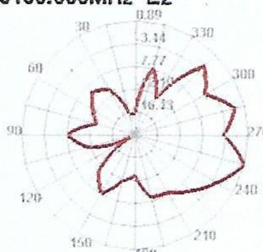
5150.000MHz E2
