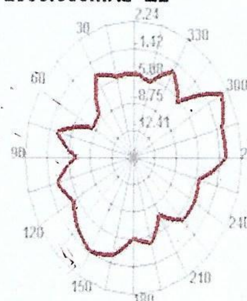
2500.000MHz E2
