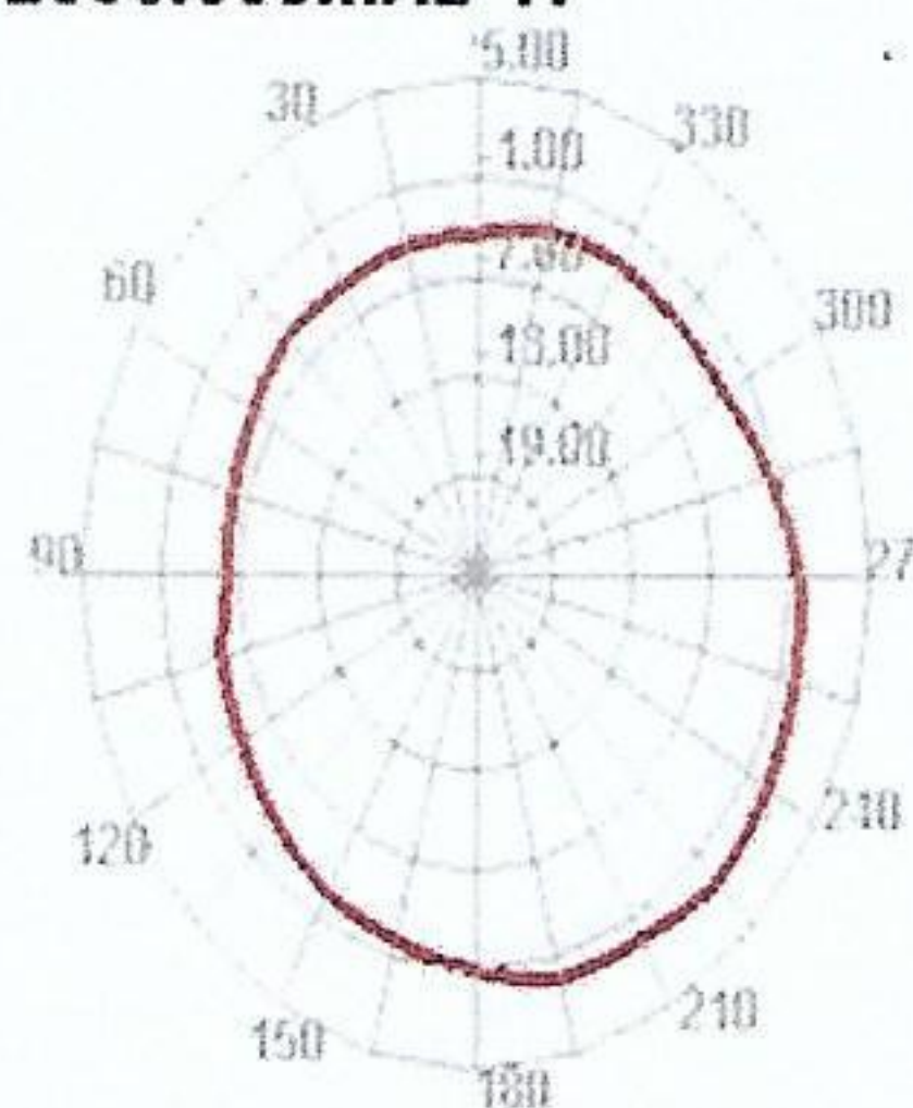
2500.000MHz H
