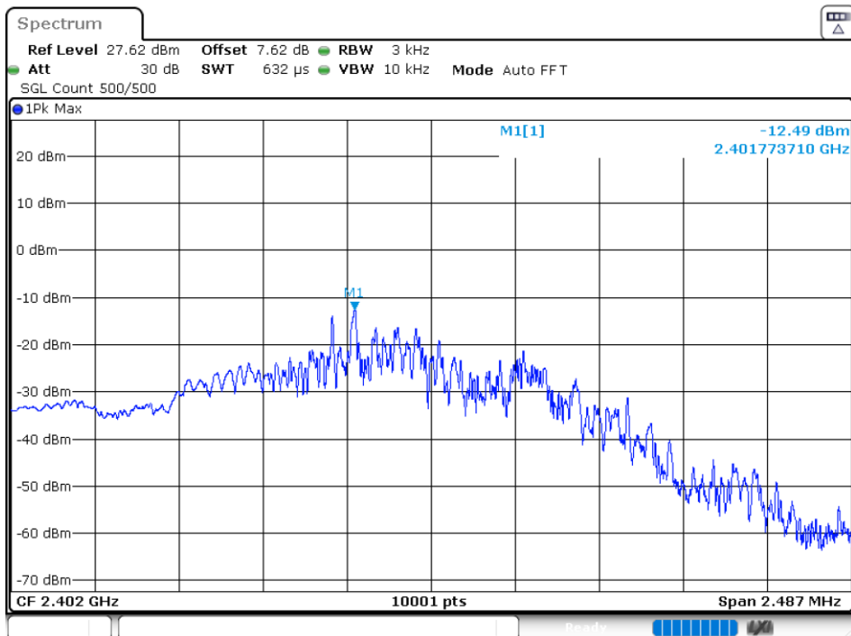
PSD NVNT 2402MHz Ant1
