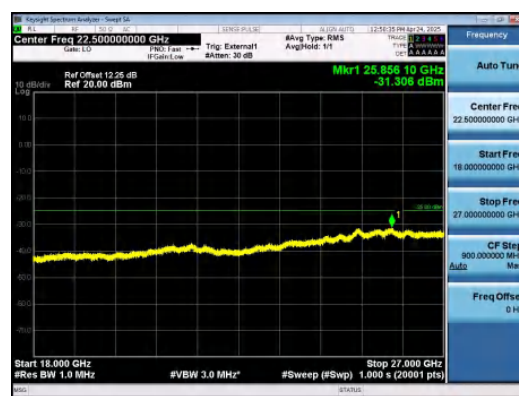
Band41-5MHz-QPSK-41565-1RB#24-18000~27 000-PASS
