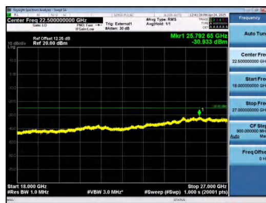
Band41-5MHz-QPSK-40620-25RB#0-18000~27 000-PASS
