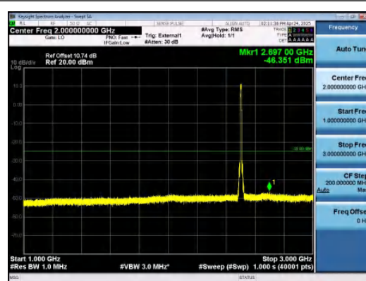
Band41-10MHz-QPSK-39700-50RB#0-1000~3000-PASS
