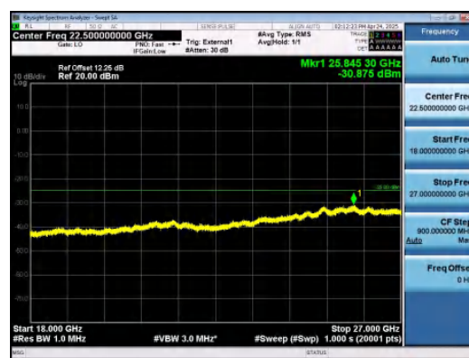
Band41-10MHz-QPSK-39700-50RB#0-18000~27000-PASS
