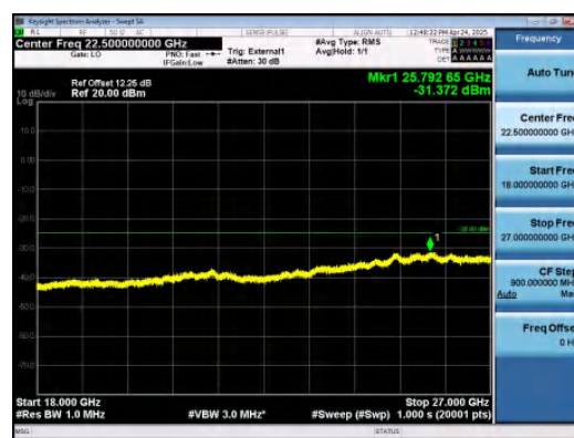
Band41-5MHz-16QAM-41565-1RB#0-18000~27 000-PASS
