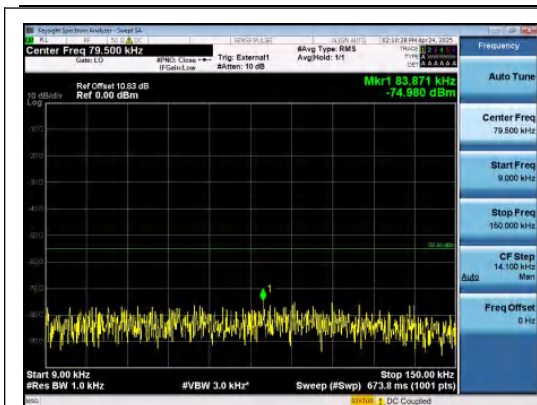
Band41-10MHz-QPSK-39700-50RB#0-0.009~0.15-PASS
