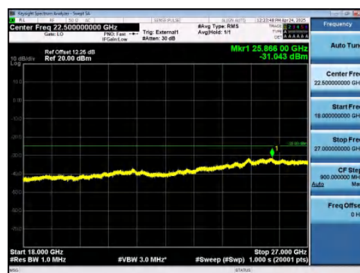
Band41-5MHz-QPSK-39675-1RB#24-18000~27 000-PASS
