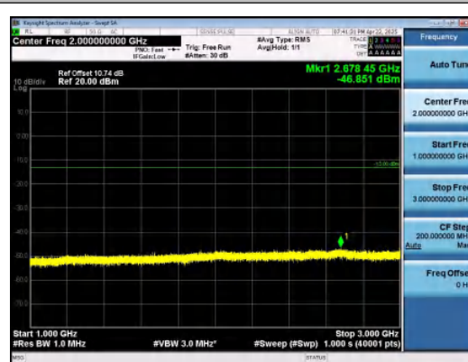
Band26(824-849)-1.4MHz-QPSK-26915-1RB#0- 1000~3000-PASS
