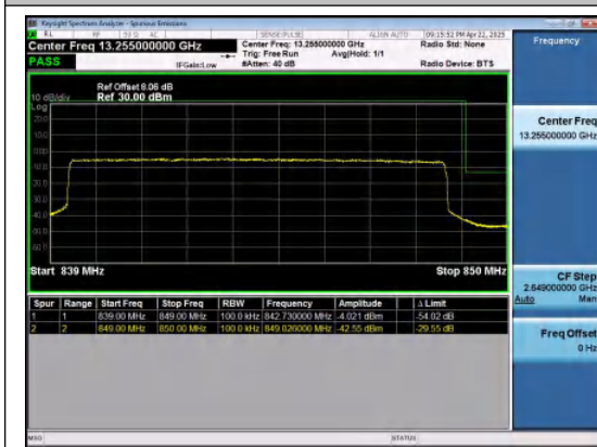
Band26(824-849)-10MHz-QPSK-26990-50RB#0-P
