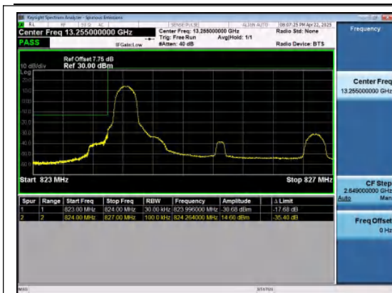
Band26(824-849)-3MHz-QPSK-26805-1RB#0-PA SS
