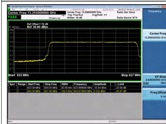
Band26(824-849)-3MHz-QPSK-26805-15RB#0-P ASS
