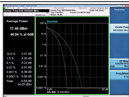
Band26(824-849)-10MHz-QPSK-26840-50RB#0-P ASS
