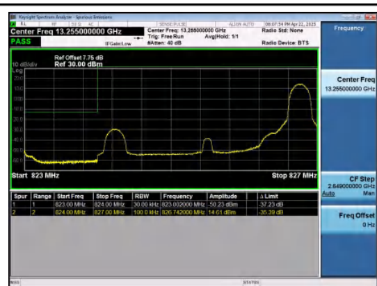
Band26(824-849)-3MHz-QPSK-26805-1RB#14-P ASS
