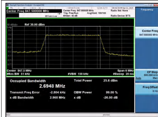
Band26(824-849)-3MHz-QPSK-27025-15RB#0-P
