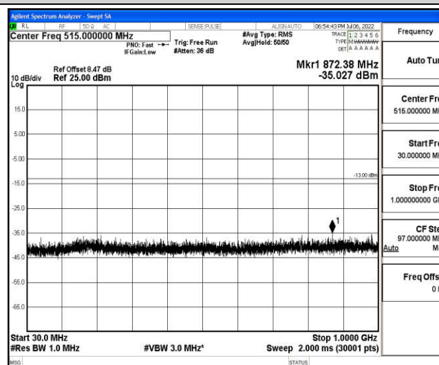
Band66-20MHz-QPSK-132322-1-0-Low-30-1000--35.03-PASS
