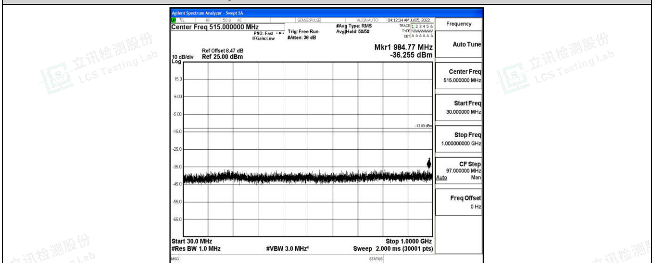
Band66-3MHz-QPSK-132322-1-0-Low-30-1000--36.26-PASS
