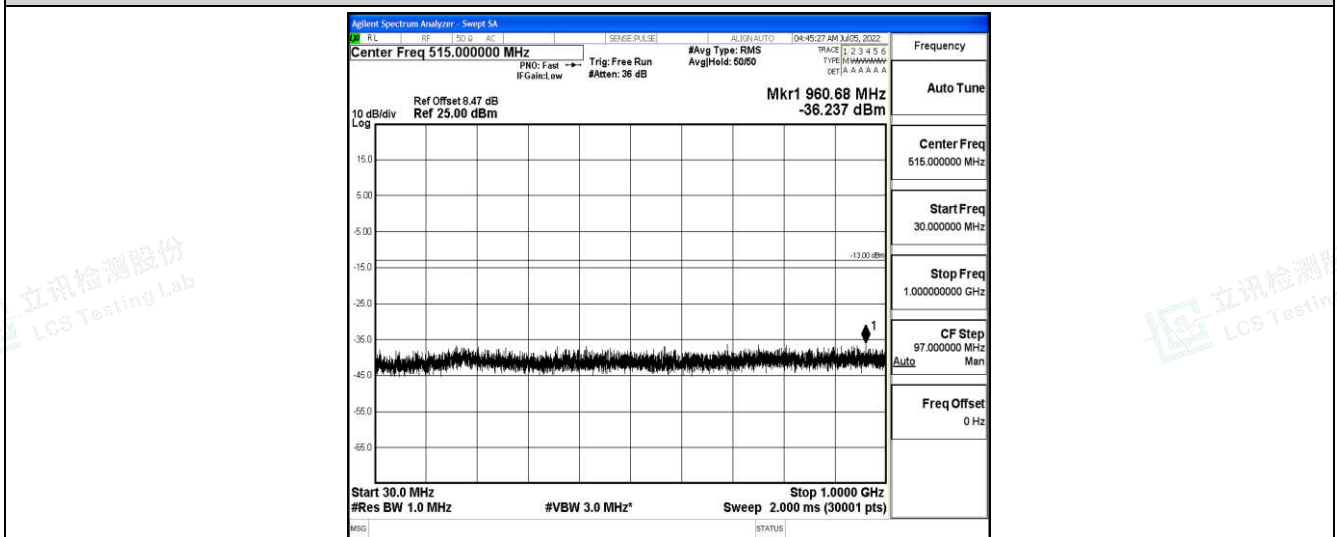
Band66-5MHz-QPSK-131997-1-0-Low-30-1000--36.24-PASS
