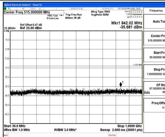
Band66-10MHz-QPSK-132022-1-0-Low-30-1000--35.68-PASS
