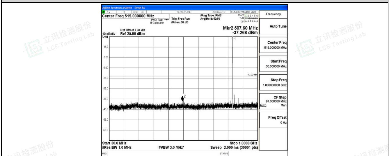
Band26-3MHz-QPSK-26915-1-0-Low-30-1000--37.27-PASS
