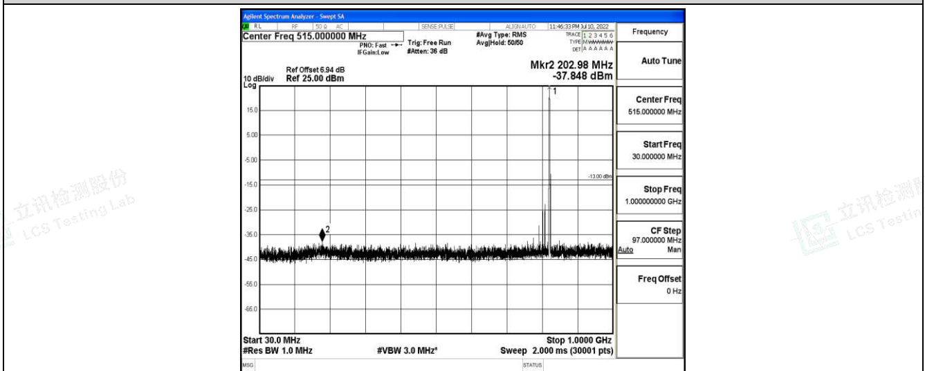
Band26-3MHz-QPSK-26805-1-0-Low-30-1000--37.85-PASS
