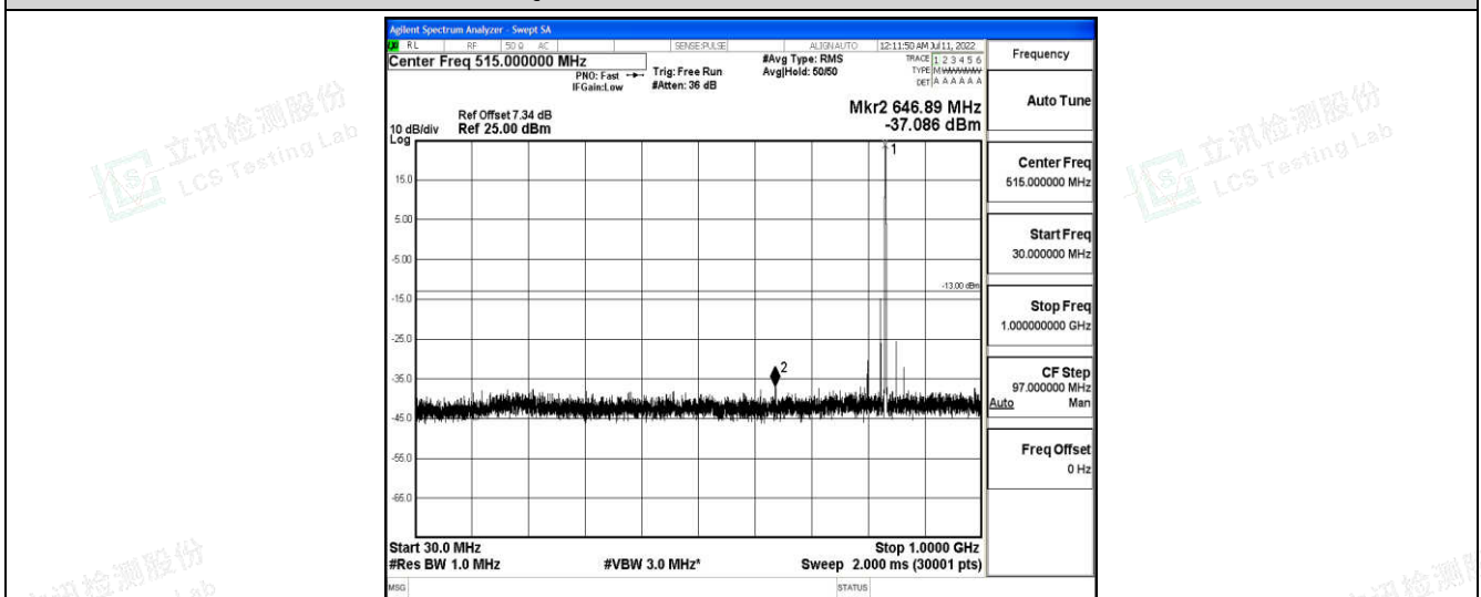
Band26-5MHz-QPSK-26915-1-0-Low-30-1000--37.09-PASS
