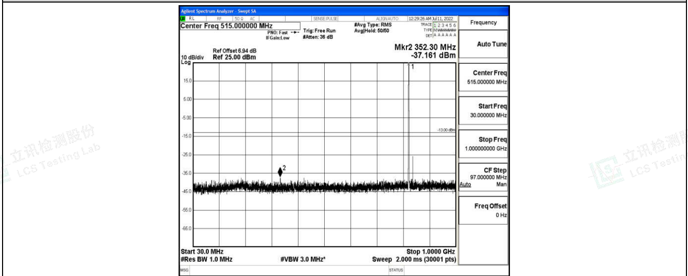
Band26-10MHz-QPSK-26840-1-0-Low-30-1000--37.16-PASS
