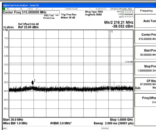
Band26-5MHz-QPSK-26740-1-0-Low-30-1000--38.03-PASS
