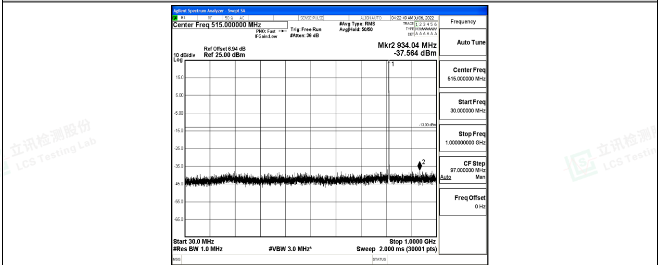
Band26-5MHz-QPSK-26715-1-0-Low-30-1000--37.56-PASS
