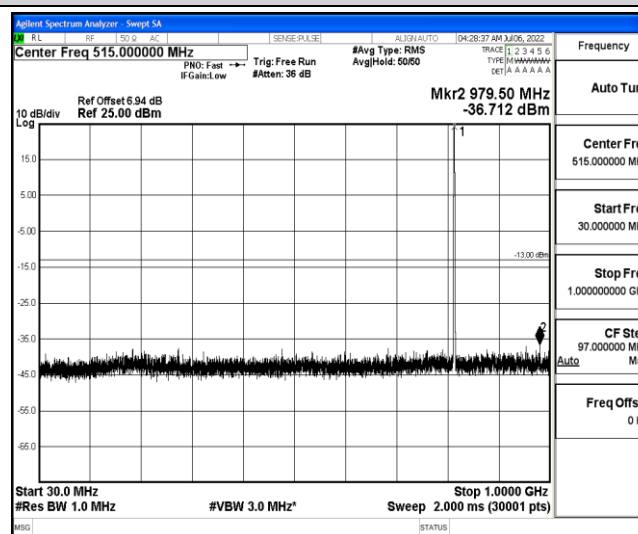
Band26-5MHz-16QAM-26740-1-0-Low-30-1000--36.71-PASS
