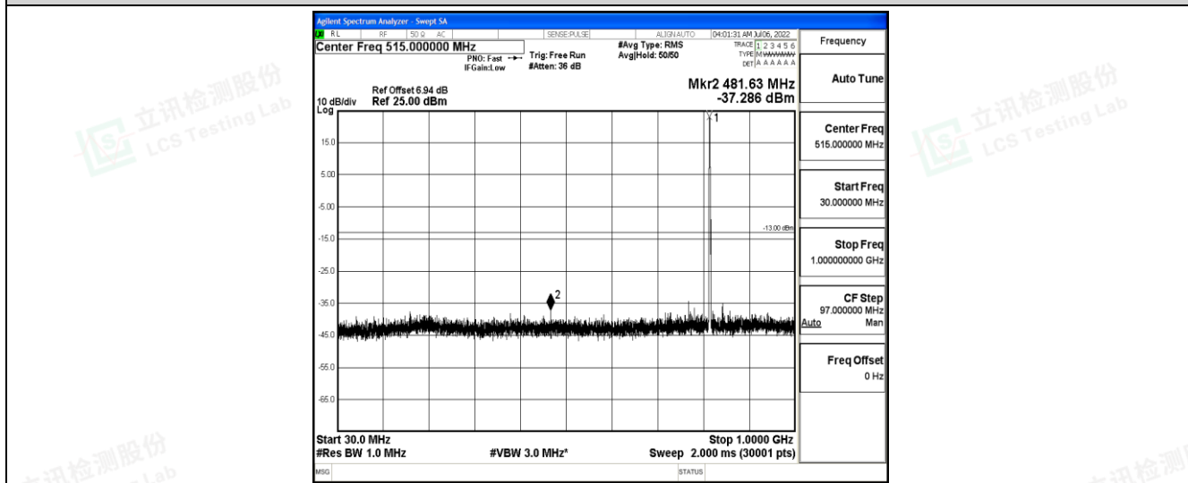
Band26-3MHz-QPSK-26740-1-0-Low-30-1000--37.29-PASS
