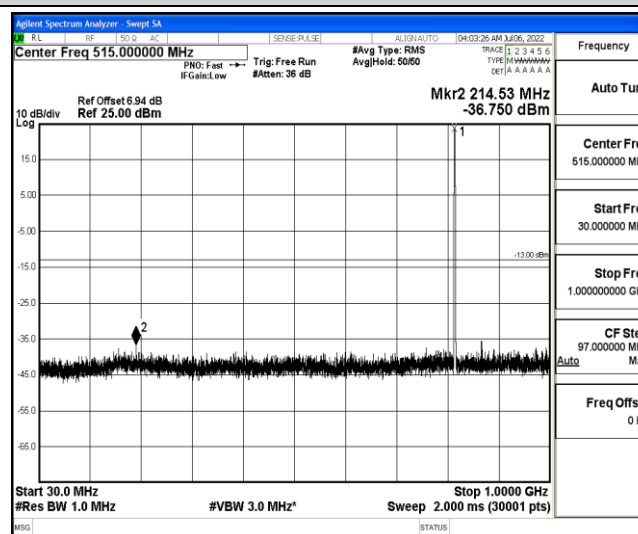
Band26-3MHz-16QAM-26740-1-0-Low-30-1000--36.75-PASS
