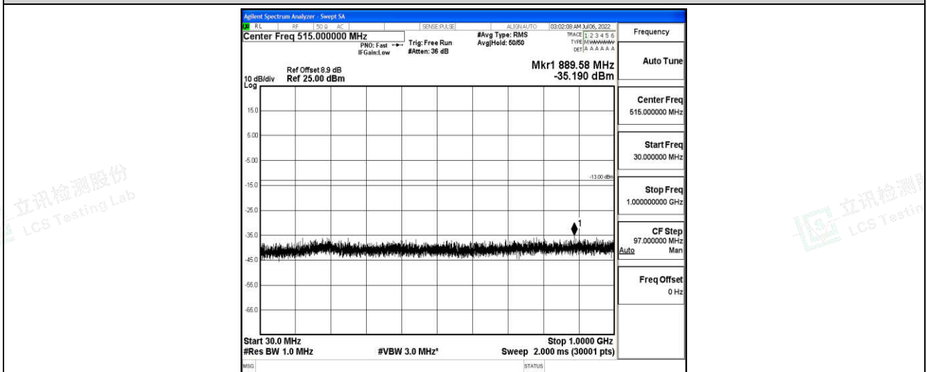
Band25-20MHz-QPSK-26140-1-0-Low-30-1000--35.19-PASS
