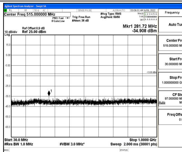
Band25-20MHz-QPSK-26365-1-0-Low-30-1000--34.91-PASS
