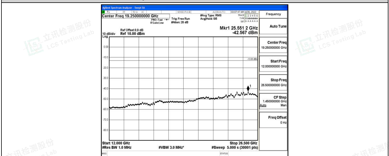
Band25-20MHz-QPSK-26365-1-0-Low-12000-26500--42.57-PASS
