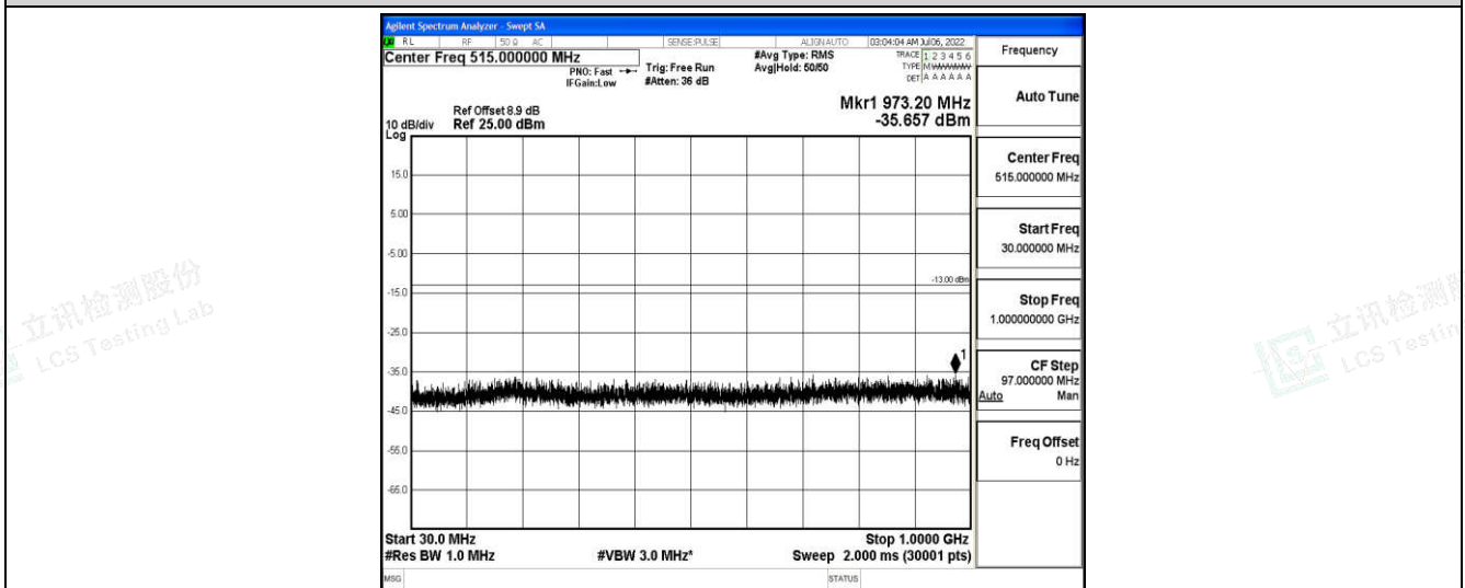
Band25-20MHz-16QAM-26140-1-0-Low-30-1000--35.66-PASS
