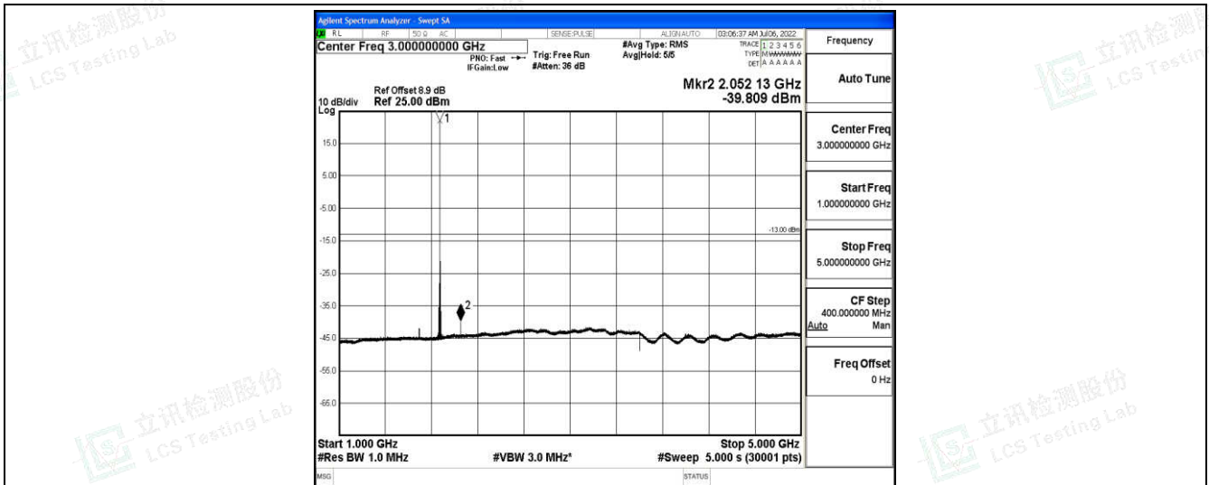
Band25-20MHz-QPSK-26365-1-0-Low-1000-5000--39.81-PASS
