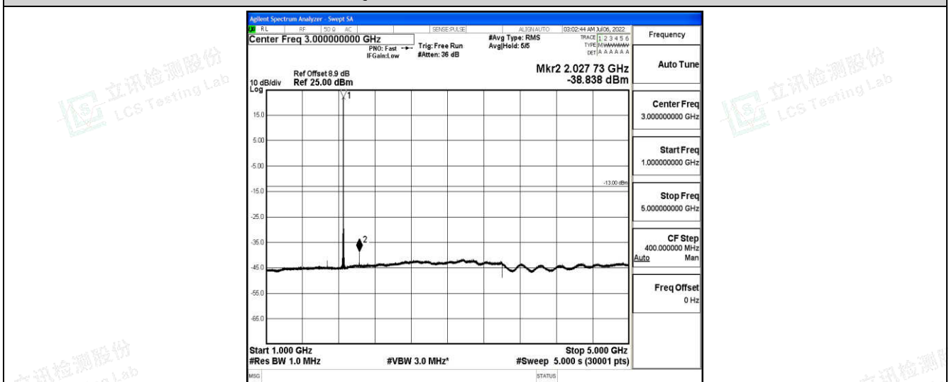
Band25-20MHz-QPSK-26140-1-0-Low-1000-5000--38.84-PASS
