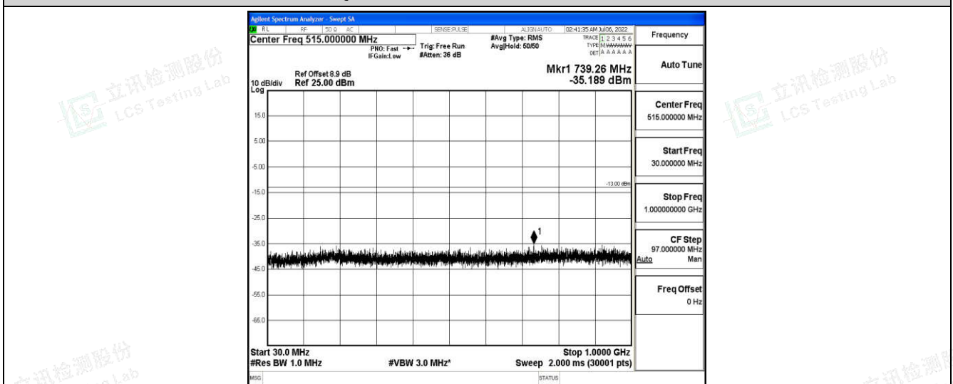
Band25-15MHz-QPSK-26365-1-0-Low-30-1000--35.19-PASS
