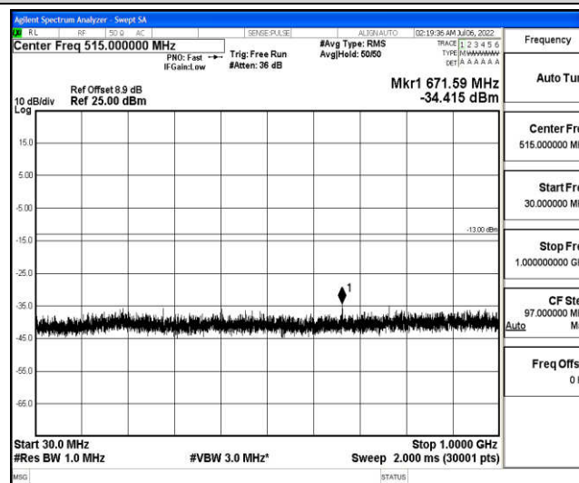
Band25-10MHz-16QAM-26365-1-0-Low-30-1000--34.42-PASS
