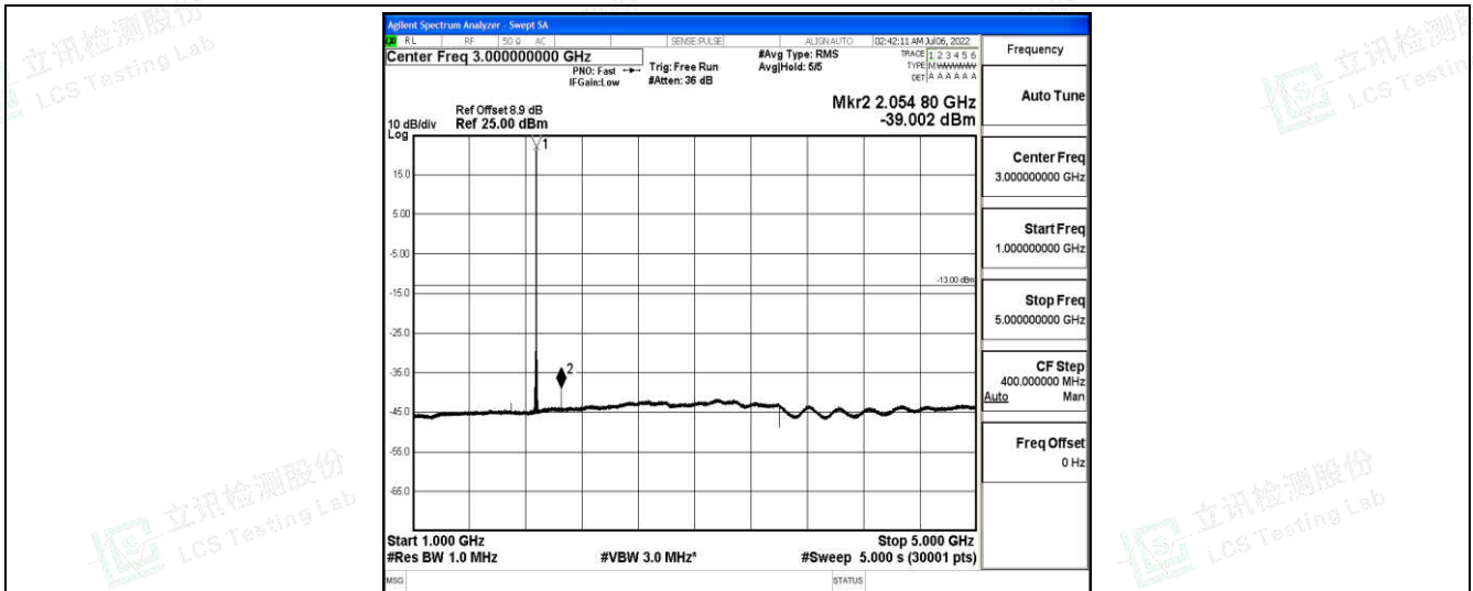
Band25-15MHz-QPSK-26365-1-0-Low-1000-5000--39-PASS
