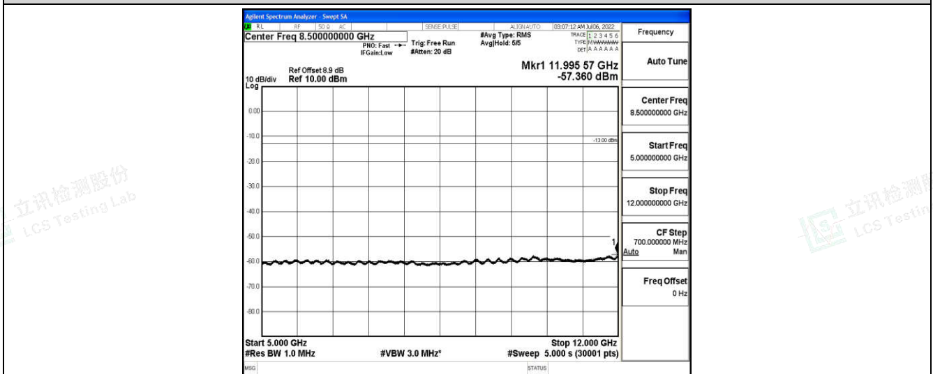
Band25-20MHz-QPSK-26365-1-0-Low-5000-12000--57.36-PASS
