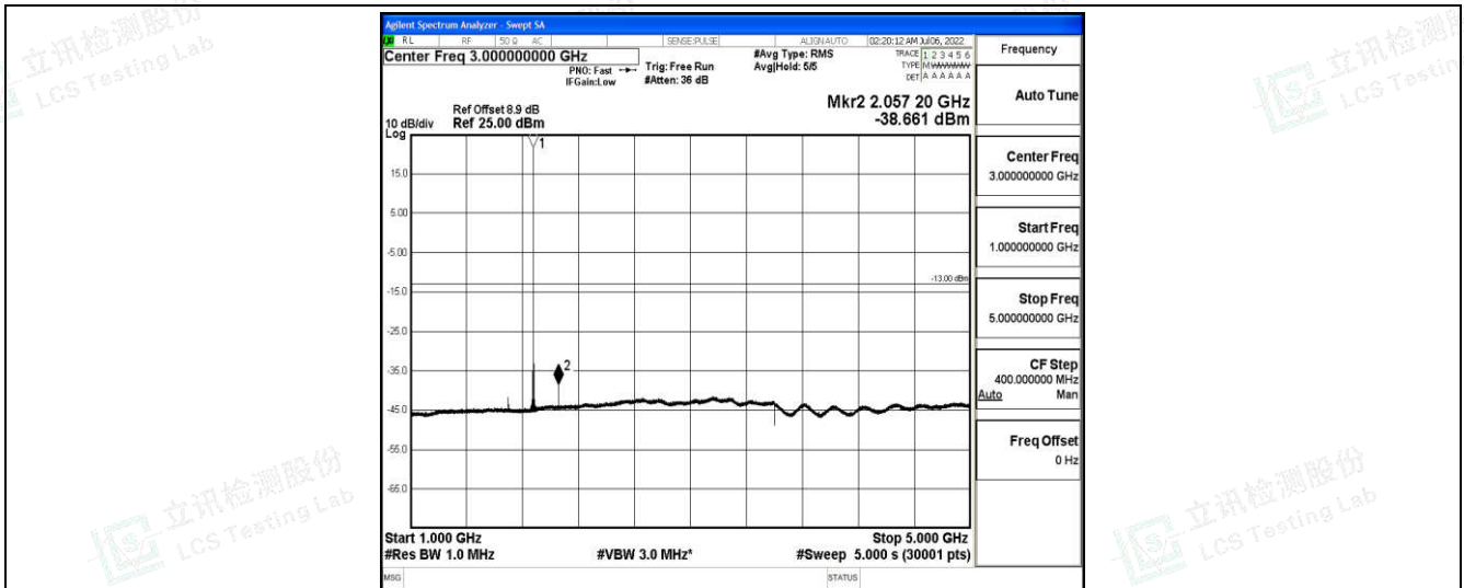
Band25-10MHz-16QAM-26365-1-0-Low-1000-5000--38.66-PASS
