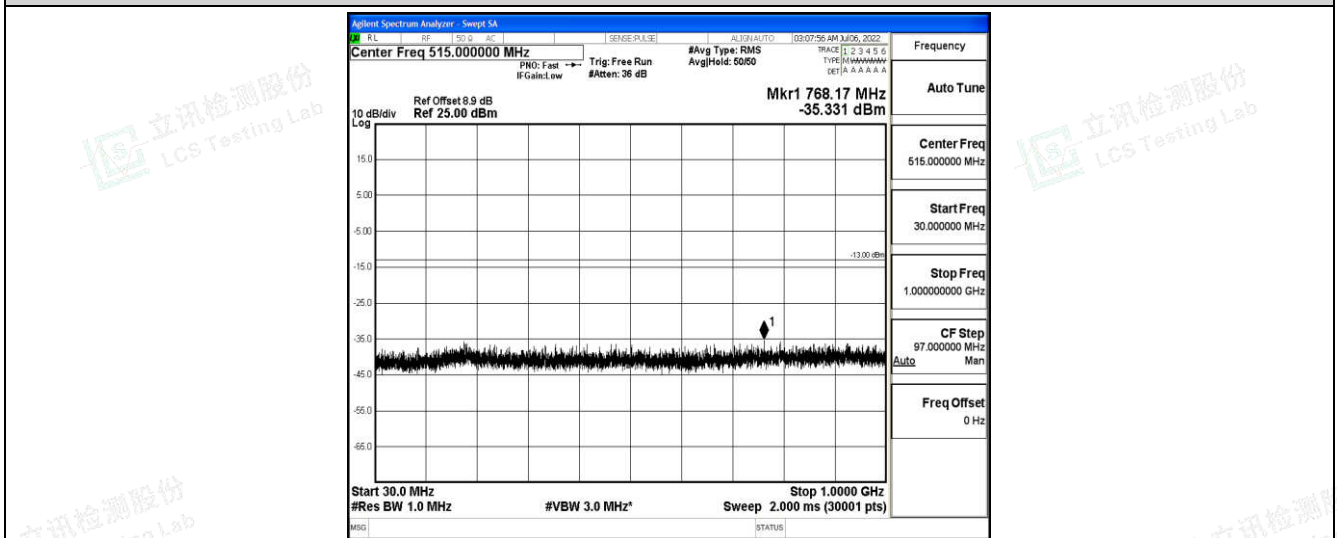
Band25-20MHz-16QAM-26365-1-0-Low-30-1000--35.33-PASS
