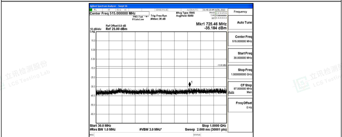
Band25-5MHz-QPSK-26065-1-0-Low-30-1000--35.18-PASS
