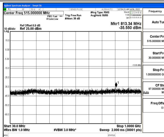
Band25-1.4MHz-QPSK-26365-1-0-Low-30-1000--35.55-PASS
