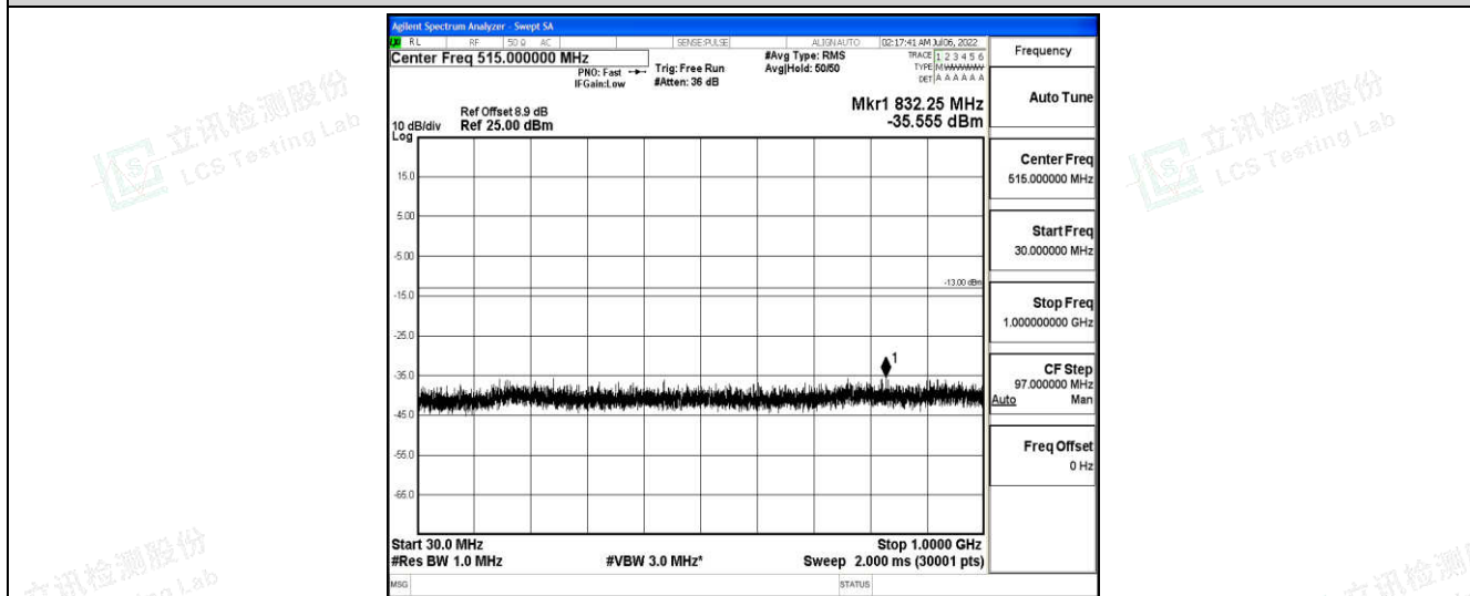
Band25-10MHz-QPSK-26365-1-0-Low-30-1000--35.56-PASS
