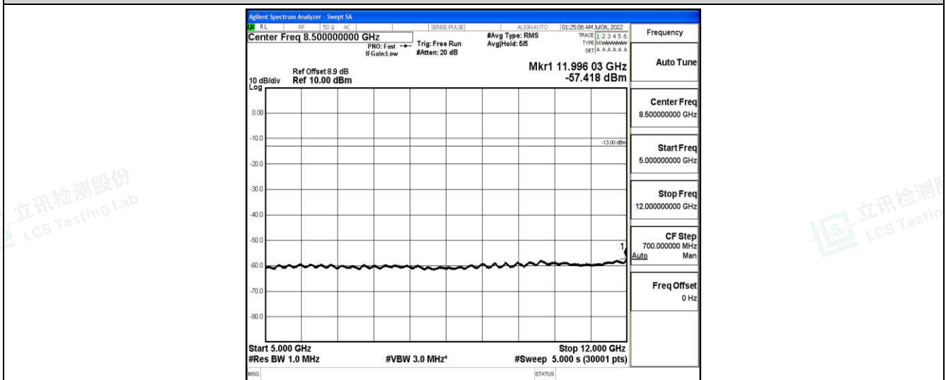
Band25-3MHz-QPSK-26365-1-0-Low-5000-12000--57.42-PASS
