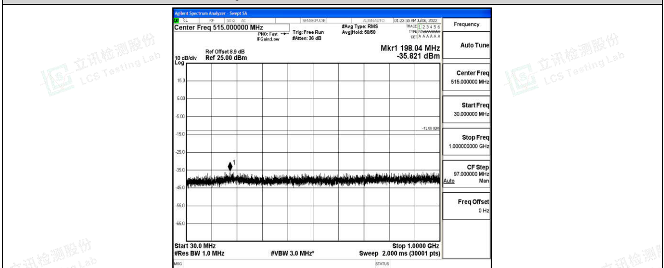
Band25-3MHz-QPSK-26365-1-0-Low-30-1000--35.82-PASS
