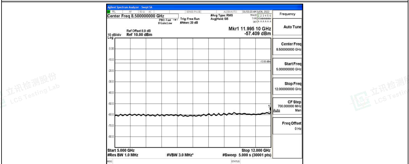
Band25-5MHz-QPSK-26365-1-0-Low-5000-12000--57.41-PASS
