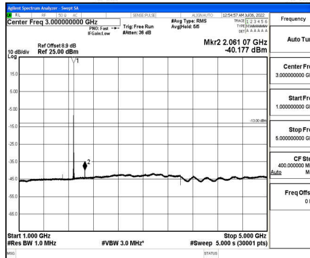
Band25-1.4MHz-QPSK-26365-1-0-Low-1000-5000--40.18-PASS
