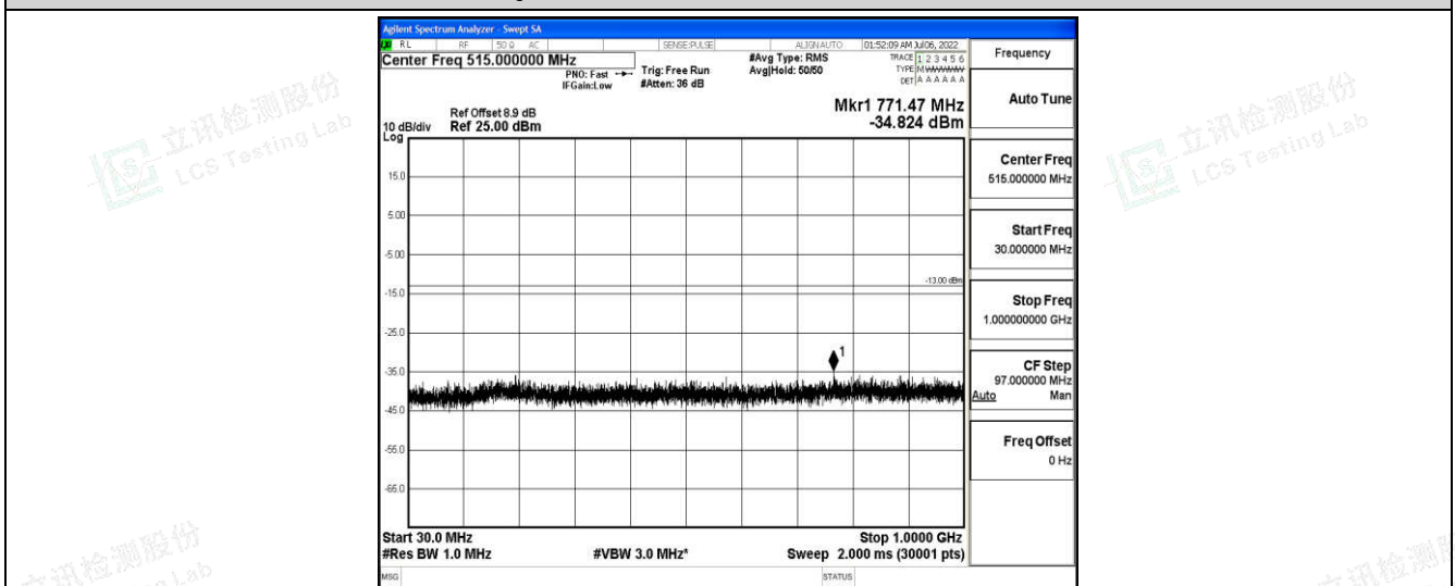
Band25-5MHz-QPSK-26365-1-0-Low-30-1000--34.82-PASS
