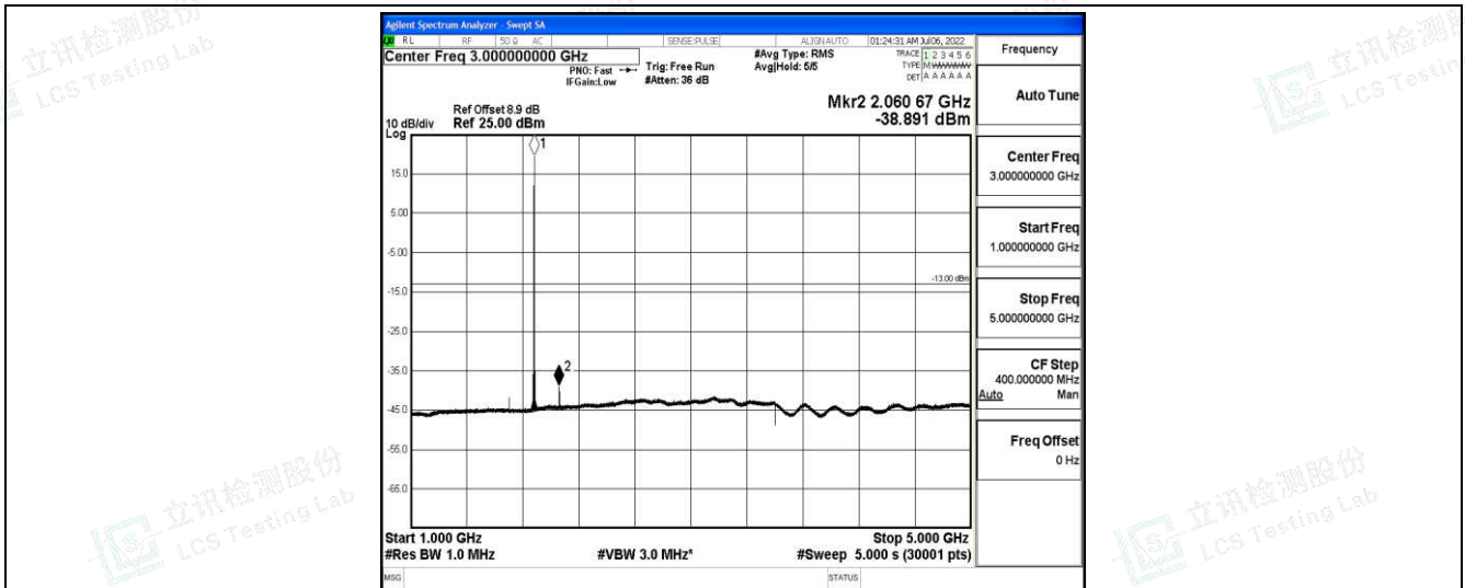
Band25-3MHz-QPSK-26365-1-0-Low-1000-5000--38.89-PASS
