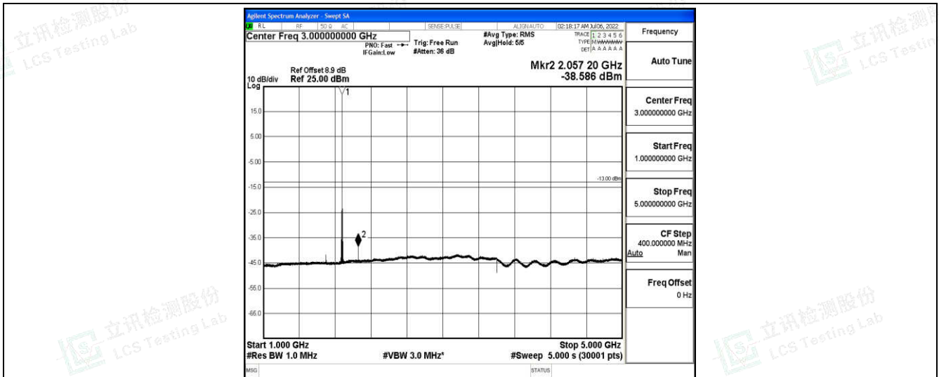
Band25-10MHz-QPSK-26365-1-0-Low-1000-5000--38.59-PASS
