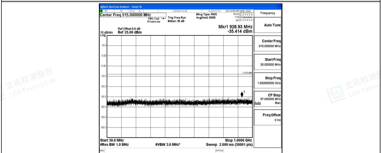
Band25-10MHz-QPSK-26090-1-0-Low-30-1000--35.41-PASS
