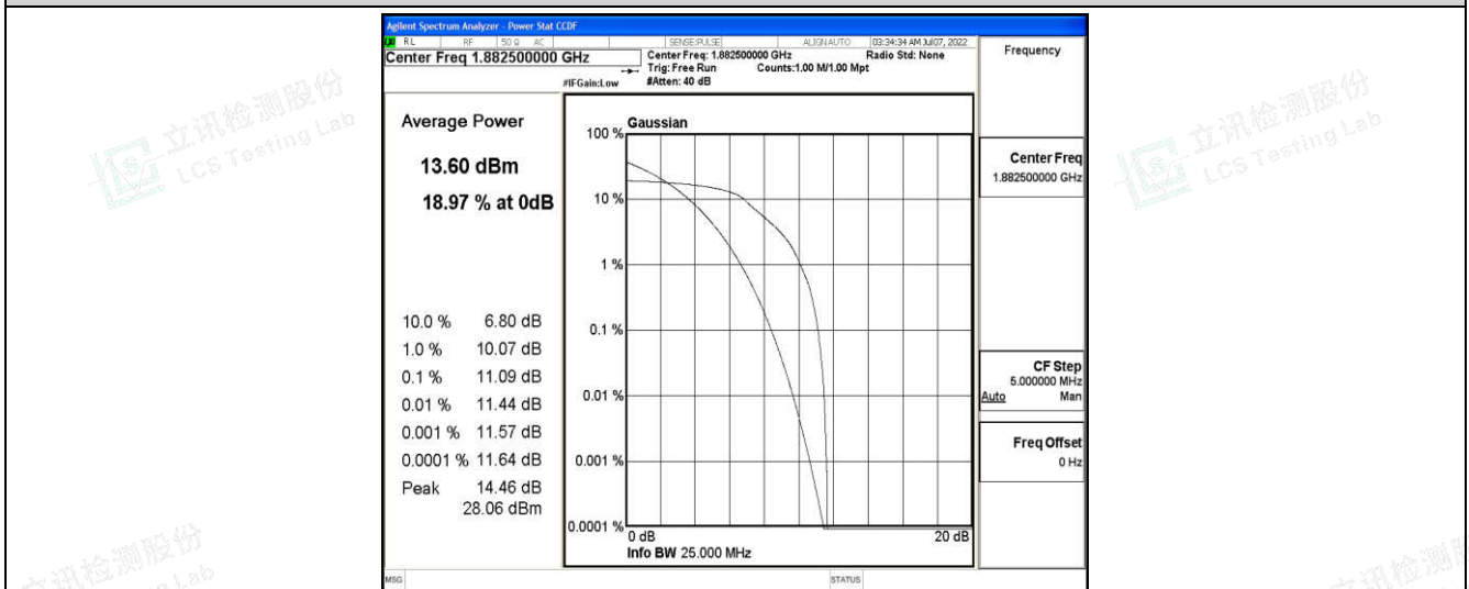
Band25-5MHz-QPSK-26365-6-0-Low-11.09-&lt;=13-PASS
