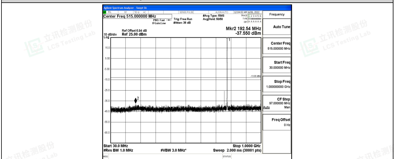
Band13-5MHz-QPSK-23230-1-0-Low-30-1000--37.55-PASS
