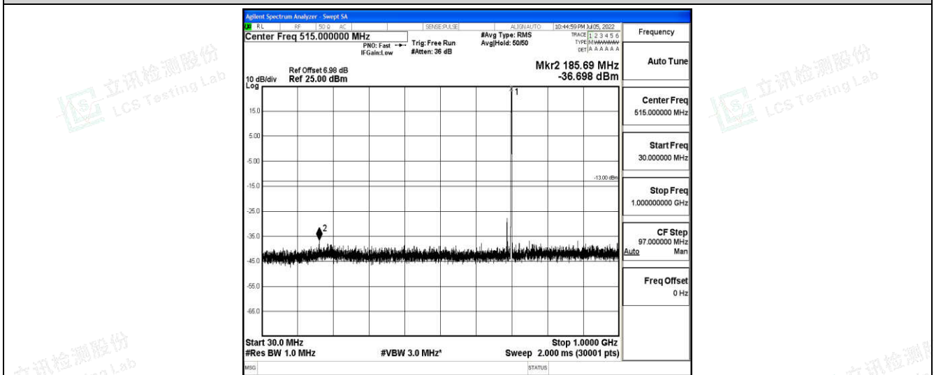
Band12-3MHz-QPSK-23095-1-0-Low-30-1000--36.7-PASS
