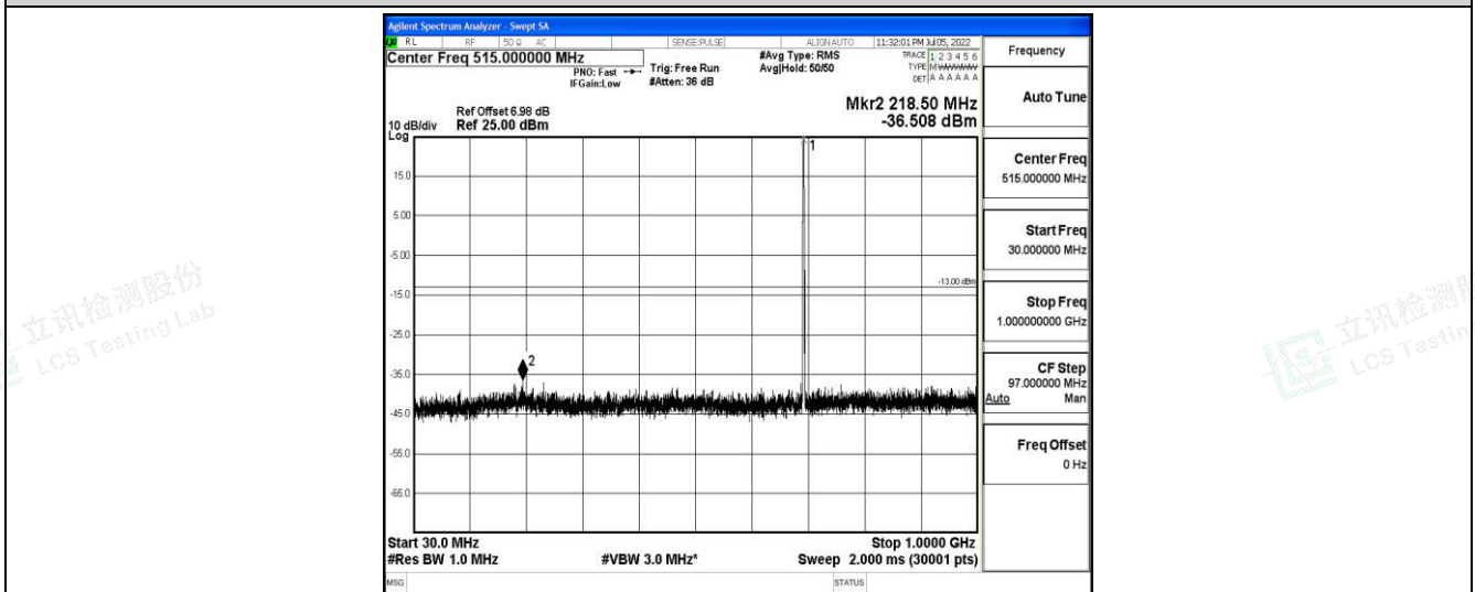
Band12-10MHz-QPSK-23060-1-0-Low-30-1000--36.51-PASS
