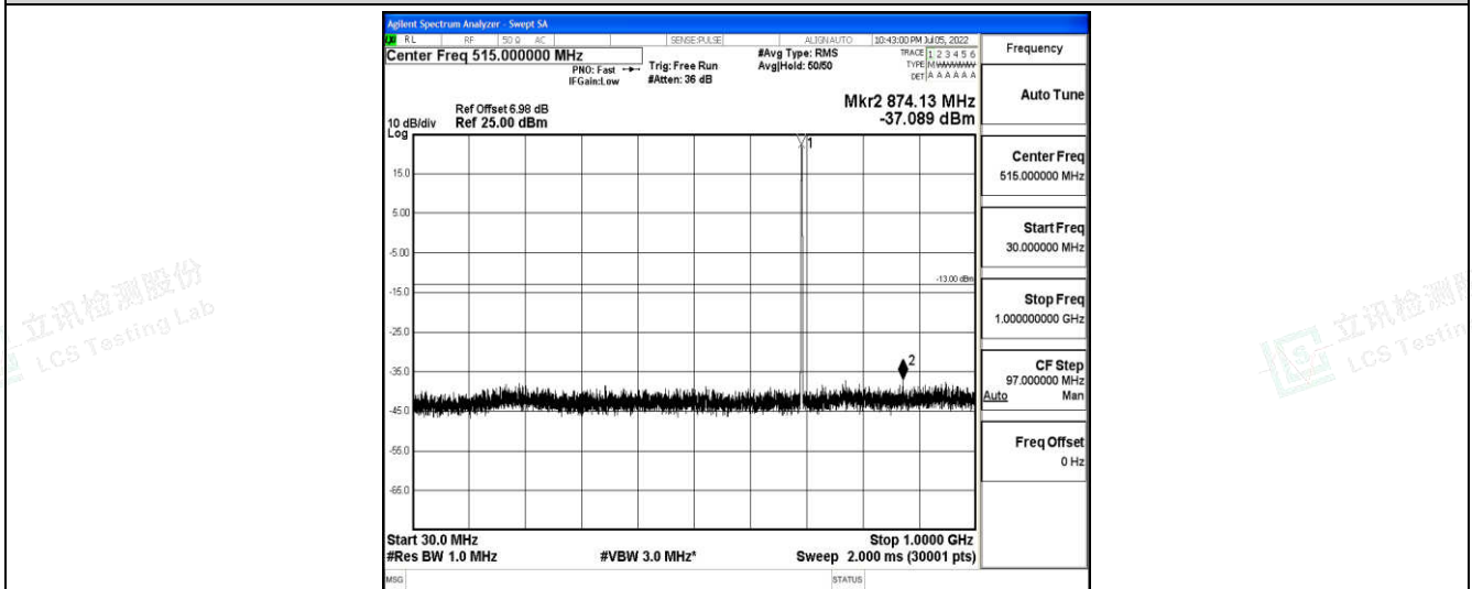
Band12-3MHz-16QAM-23025-1-0-Low-30-1000--37.09-PASS
