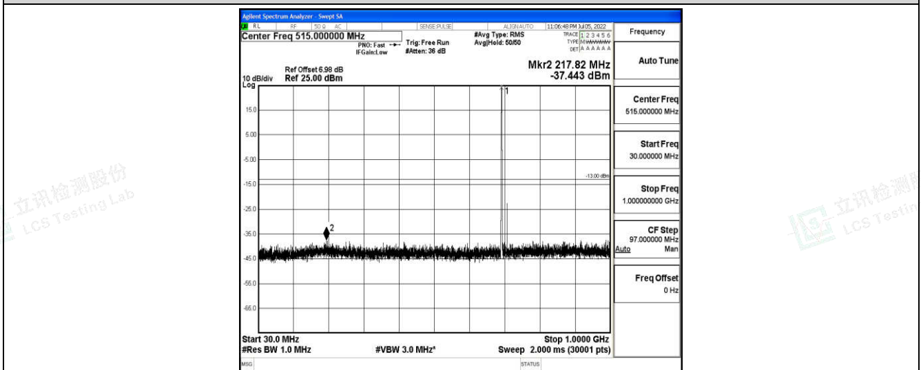
Band12-5MHz-QPSK-23035-1-0-Low-30-1000--37.44-PASS
