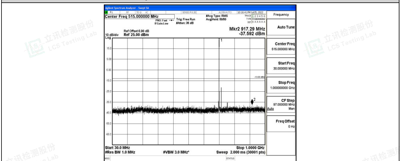
Band12-1.4MHz-QPSK-23095-1-0-Low-30-1000--37.59-PASS
