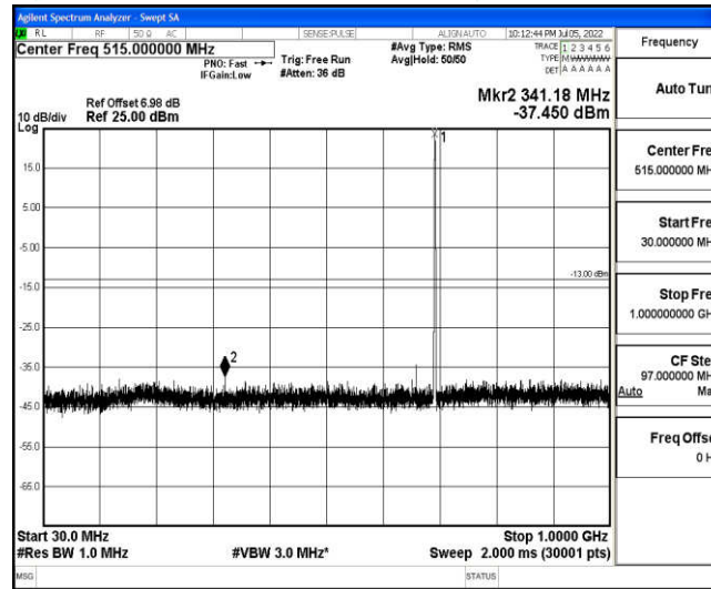
Band12-1.4MHz-QPSK-23017-1-0-Low-30-1000--37.45-PASS
