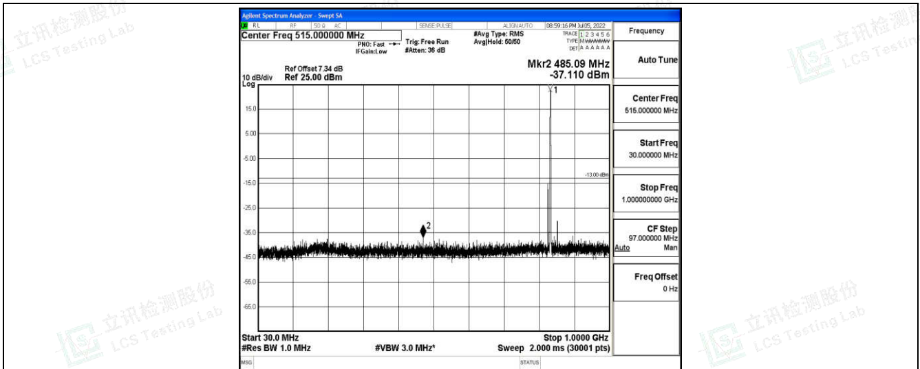
Band5-3MHz-QPSK-20525-1-0-Low-30-1000--37.11-PASS
