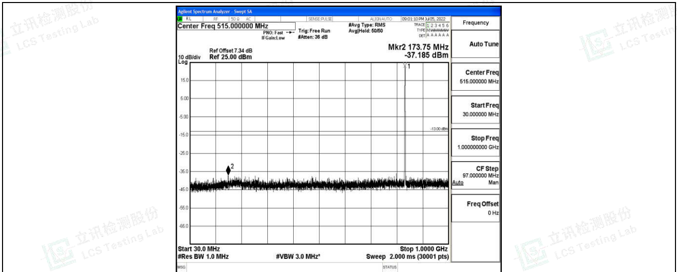
Band5-3MHz-16QAM-20525-1-0-Low-30-1000--37.19-PASS
