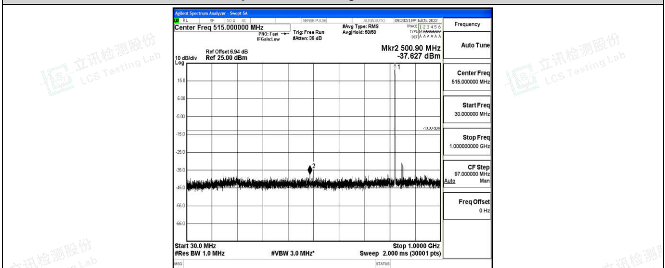
Band5-5MHz-QPSK-20425-1-0-Low-30-1000--37.63-PASS
