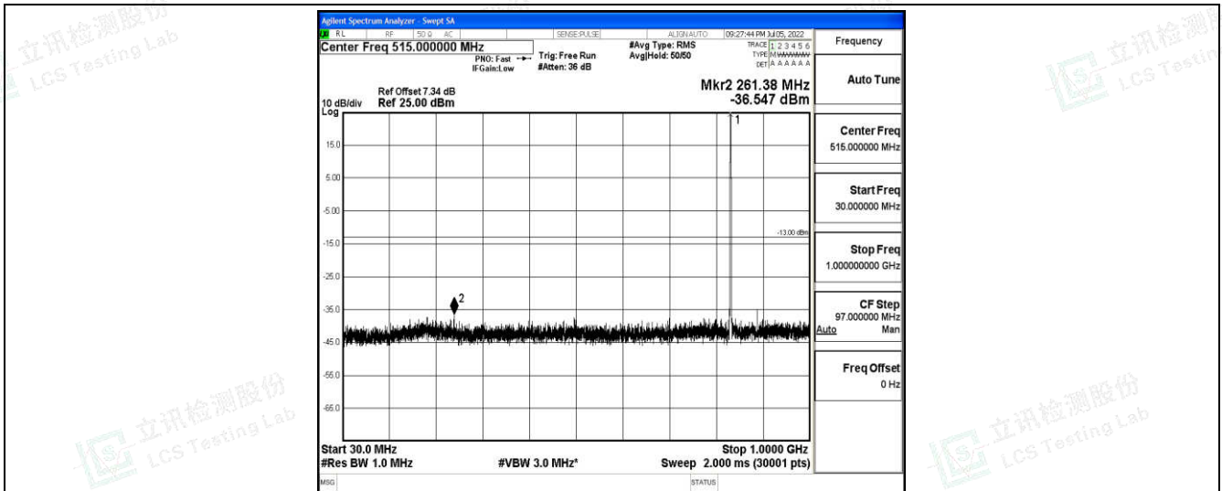
Band5-5MHz-QPSK-20525-1-0-Low-30-1000--36.55-PASS
