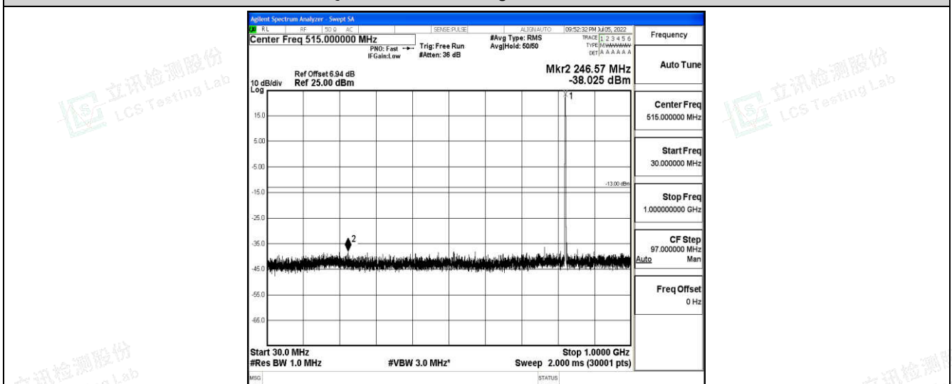
Band5-10MHz-16QAM-20450-1-0-Low-30-1000--38.03-PASS
