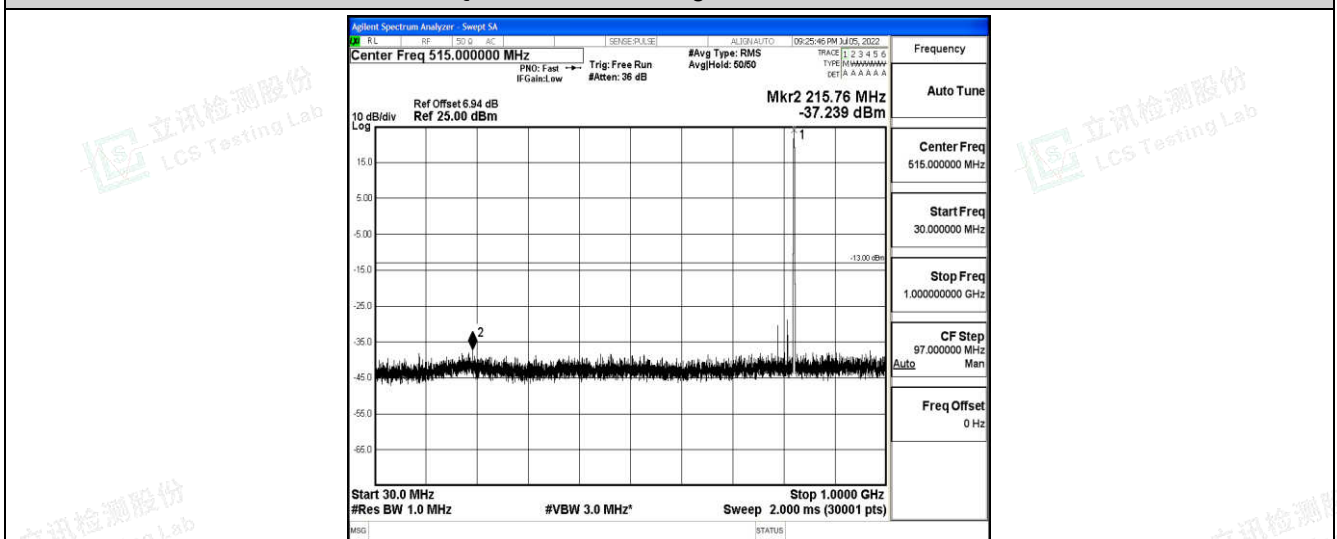
Band5-5MHz-16QAM-20425-1-0-Low-30-1000--37.24-PASS
