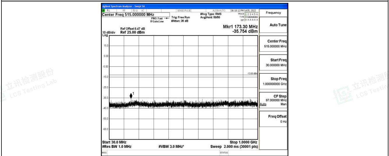
Band4-10MHz-QPSK-20000-1-0-Low-30-1000--35.75-PASS
