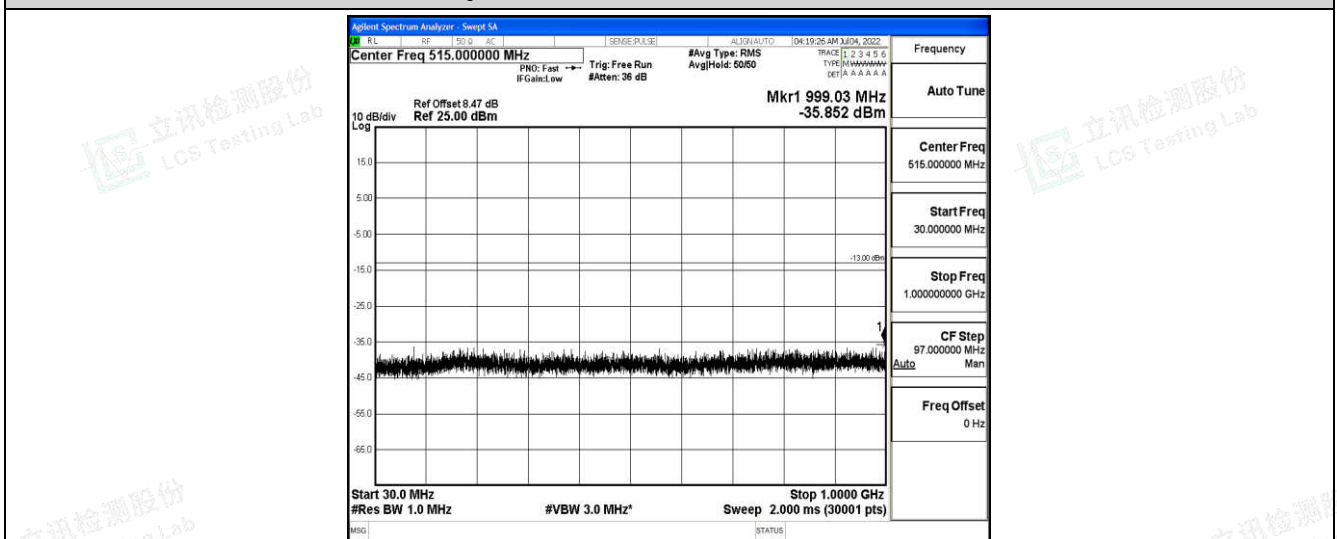
Band4-3MHz-QPSK-20175-1-0-Low-30-1000--35.85-PASS
