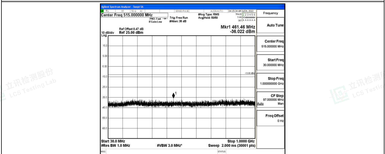
Band4-3MHz-QPSK-19965-1-0-Low-30-1000--36.02-PASS
