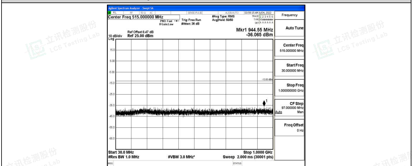
Band4-1.4MHz-QPSK-20175-1-0-Low-30-1000--36.07-PASS
