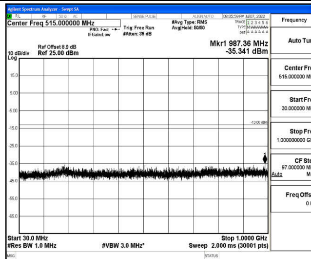
Band2-20MHz-QPSK-18700-1-0-Low-30-1000--35.34-PASS
