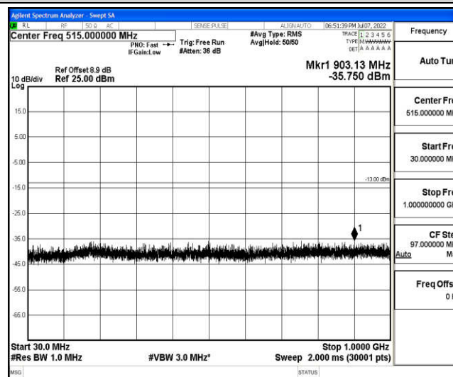
Band2-5MHz-QPSK-18900-1-0-Low-30-1000--35.75-PASS
