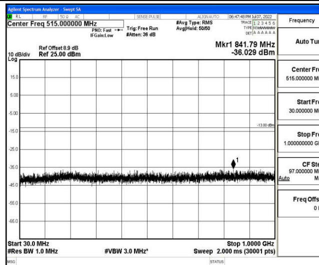
Band2-5MHz-QPSK-18625-1-0-Low-30-1000--36.03-PASS
