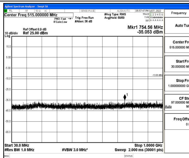
Band2-1.4MHz-QPSK-18900-1-0-Low-30-1000--35.05-PASS
