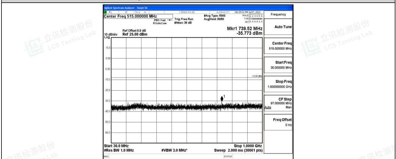
Band2-3MHz-QPSK-18900-1-0-Low-30-1000--35.77-PASS
