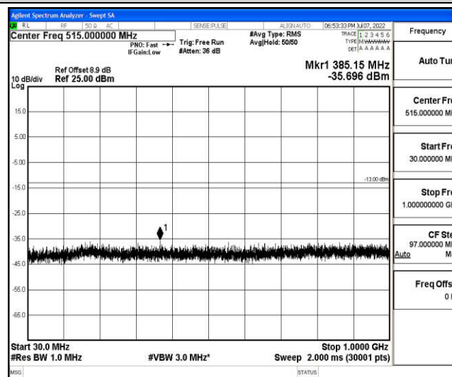
Band2-5MHz-16QAM-18900-1-0-Low-30-1000--35.7-PASS
