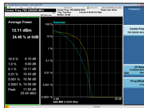
B13-5M-Mid CH-PAPR-Q16
