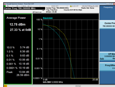
B13-5M-Mid CH-PAPR-QPSK
