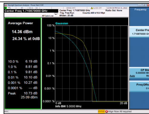
B4-3M-Low CH-PAPR-QPSK
