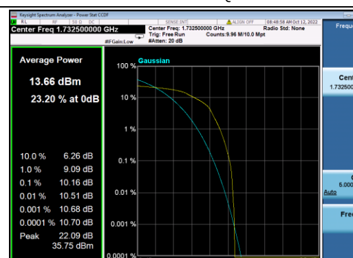
B4-1.4M-Mid CH-PAPR-Q16
