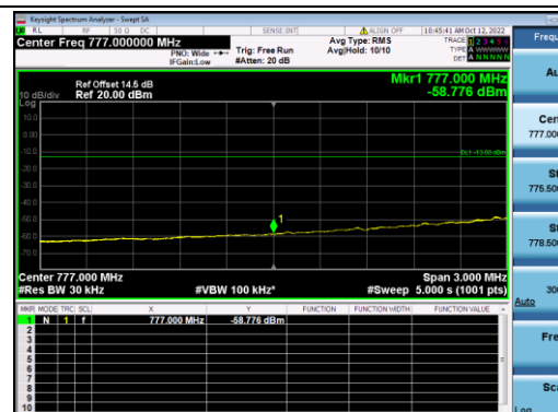
B13-5M-Low CH-BE-Q16-Full RB 0
