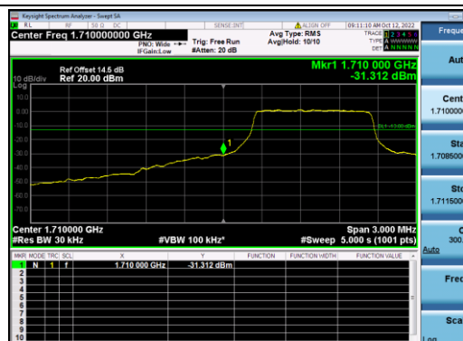
B4-5M-Low CH-BE-Q16-Full RB 0
